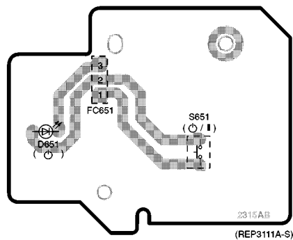
C SWITCH P.C.B.
