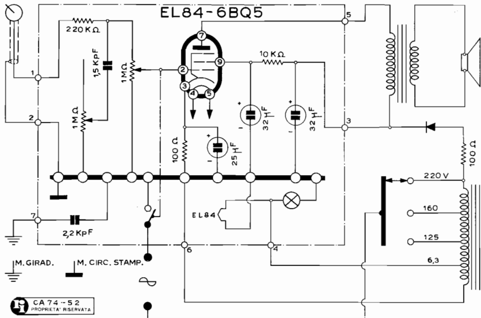
LESA - Fonovaligia Mod. Lesaphon 210 "Biadix,,
