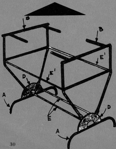
Fig. 2 Il telaio è costruito interamente in tondino di ferro di due misure diverse, facilmente acquistabile, per coloro che non avessero rinvenuto il vecchio porta-bagagli, presso qualsiasi negozio di ferramenta.
