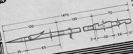
Fig. 2 - Piastrina con mirino applicata nella parte anteriore della canna; il foro centrale superiore serve come guida alla corsa della freccia; ai due fori laterali vengono fissati gli elastici.
