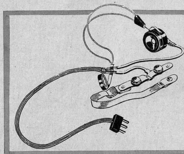
Fig. 4 - I componenti che accompagnano il pescatore subacqueo in immersione sono il laringofono e l'auricolare. Il collegamento con chi sta in emersione è costituito da un cavo di gomma o plastica a tre fili. Le saldature sono ricoperte con nastro isolante comune. Fig. 5 - Il laringofono e la cuffia, che accompagnano il pescatore subacqueo, sono collegati tra loro e al cavo che fa capo alla spina, nel modo indicato in figura. Un conduttore della cuffia e uno del laringofono sono uniti tra di loro e al filo di massa (2).
