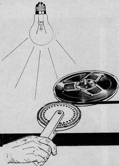
Fig. 2 - Per il controllo della velocità di trascinamento del nastro magnetico in un magnetofono occorre esercitare una leggera pressione col disco stroboscopico sul nastro contenuto nella bobina. La sorgente luminosa potrà essere quella di una lampada alimentata dalla corrente alternata della rete-luce. Se la velocità di trascinamento del nastro è esatta, i trattini della circonferenza dello stroboscopio, corrispondenti alla velocità in esame, dovranno apparire fermi.
