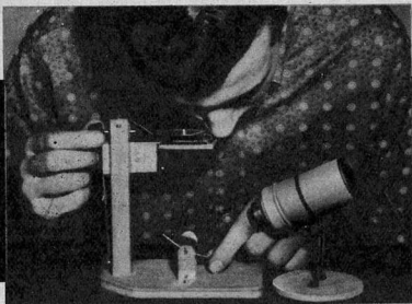
Fig. 1 - Il microscopio è costituito da due parti principali in legno: il basamento e la colonna di sostegno. Sul basamento sono fissati i supporti per lo specchietto riflettente mentre sulla colonna sono sistemati il supporto fisso per la lente alla glicerina e lo scorrevole porta-vetrino. Mediante il sistema formato dalla manopola, dal filo di nailon e dall'elastico, sono possibili i piccoli spostamenti del vetrino porta-oggetti per l'esatta messa a fuoco.
