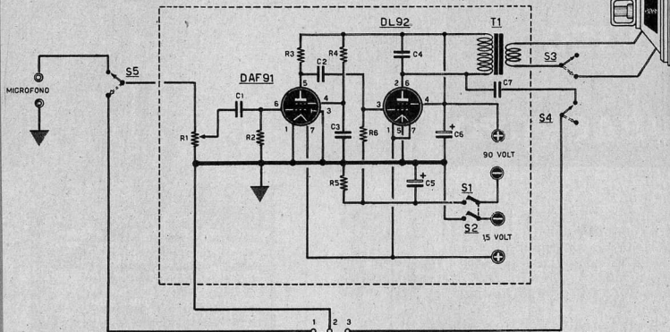
Fig. 2 - Schema elettrico dell'interfono.
