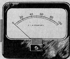
Fig. 2 - Vista frontale dello strumento da 100 microampere fondo-scala impiegato per la realizzazione del termometro a transistor.
