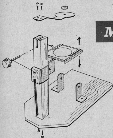
Fig. 1 - Il microscopio è costituito da due parti principali in legno: il basamento e la colonna di sostegno. Sul basamento sono fissati i supporti per lo specchietto riflettente mentre sulla colonna sono sistemati il supporto fisso per la lente alla glicerina e lo scorrevole porta-vetrino. Mediante il sistema formato dalla manopola, dal filo di nailon e dall'elastico, sono possibili i piccoli spostamenti del vetrino porta-oggetti per l'esatta messa a fuoco.
