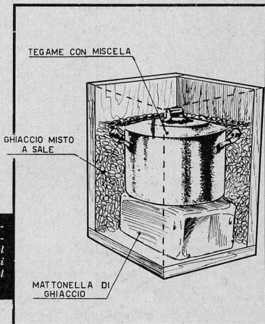
Fig.1 - La gelatiera è costituita da una cassettona di legno dentro alla quale viene posto il recipiente contenente la miscela da congelare. Nel fondo si pone un pezzo di ghiaccio intero e poi tutto attorno, ed anche sopra il coperchio, del ghiaccio tritato mescolato a sale.
