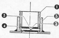
Fig. 13 - Altro sistema di tenuta obblò.
