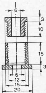
Fig. 17 - Altro tipo di premistoppa.
