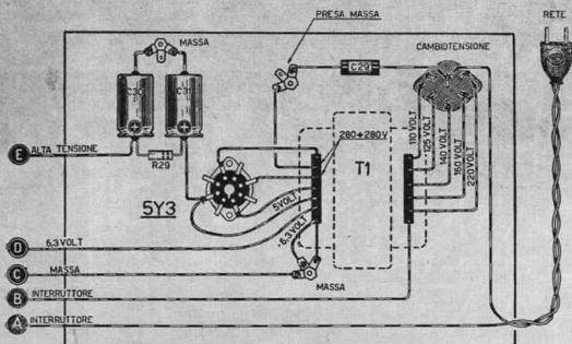
N. B. — Collegare le posizioni contrassegnate con le lettere A-B-C-D-E con le corrispondenti del ricevitore di cui a figura 3.
