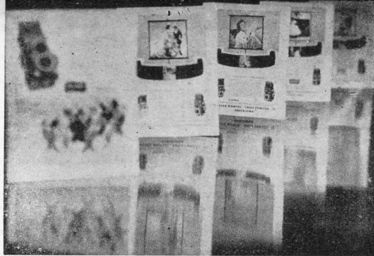
Fig. 8 - Sistemando giornali a distanze diverse, saremo in grado di controllare, oltre alla profondità di campo, l'esattezza del telemetro. Nella foto è possibile constatare come il centro risulti a fuoco.
