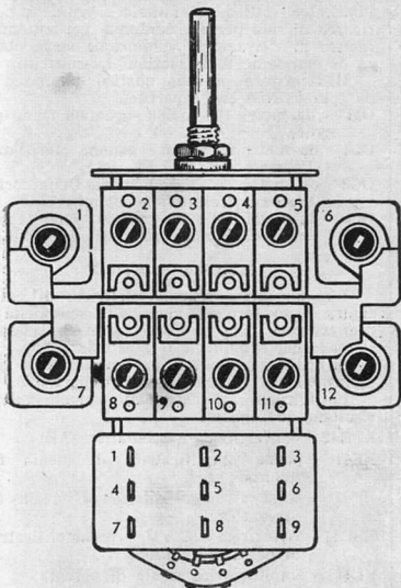
Fig. 2 - Gruppo A. F. CS41-bis della Corbetta.
