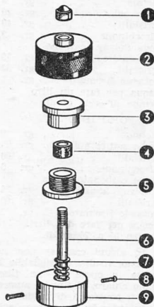
Fig. 4 - Scomposizione dispositivo ricarica a pomello: 1) dado cieco di ritagno; 2) pomello esterno zigrinato di ricarica; 3) ghiera superiore premistoppa; 4) amianto; 5) ghiera inferiore premistoppa; 6) perno; 7) molla; 8) viti serraggio; 9) ghiera incastolamento pomello macchina.
