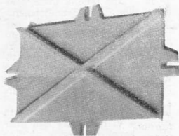
Fig. 21 - Coperchio rinforzato a mezzo costolature.
