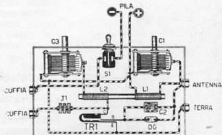
Fig. 2 - SCHEMA PRATICO
