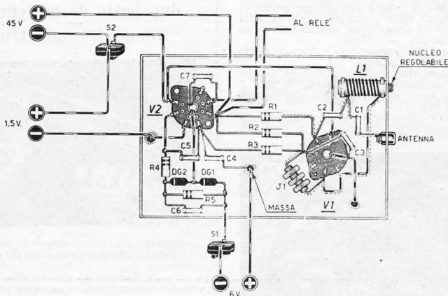
Fig. 3 - Schema pratico.
