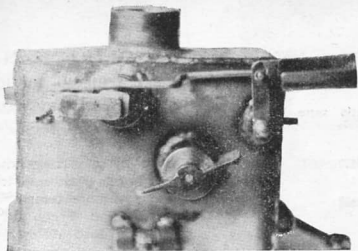
Fig. 23 - Vista di fianco di una camera stagna.
