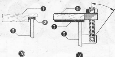
Fig. 9 - Il coperchio della camera stagna dovrà risultare serrato a tenuta a mezzo guarnizione in gomma e bullone incernierato all'estremità filettata. A - 1) coperchio; 2) guarnizione in gomma; 3) parete camera. B - 1) coperchio; 2) guarnizione in gomma; 3) parete camera.
