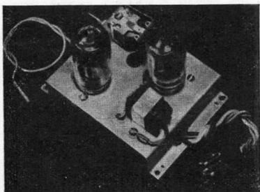
Fig. 4 - Sistemazione dei componenti che risultano montati sulla parte superiore del telaio.
