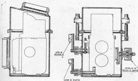
Fig. 19 - Camera stagna per macchina tipo Rollei sezionata.
