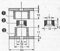
Fig. 16 - Tipo di premistoppa.
