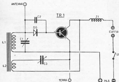
Fig. 1 - SCHEMA ELETTRICO
