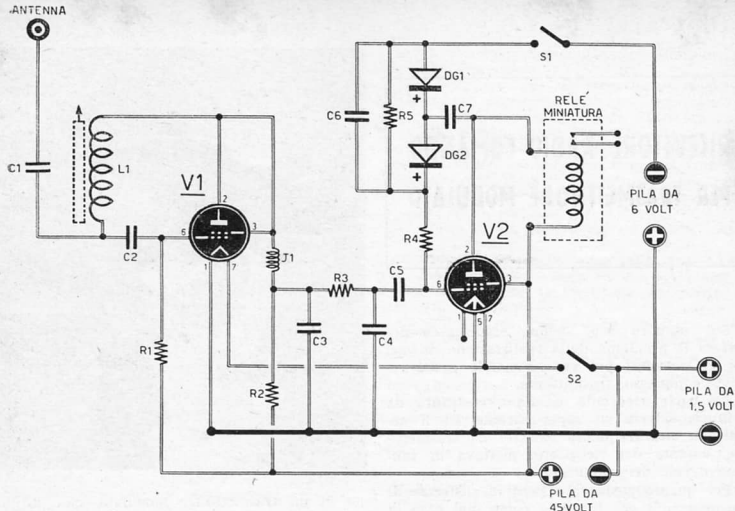
Fig. 1 - Schema elettrico
