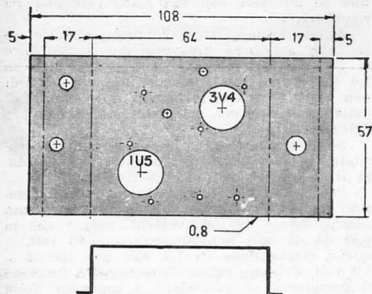
Fig. 2 - Dimensionamento telaio metallico.
