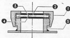
Fig. 14 - Dal punto di vista estetico il sistema di tenuta obblò esemplificato a figura risulta essere senza meno il preferibile.
