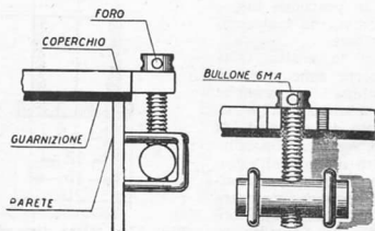
Fig. 10 - Sistema di aggancio e tenuta coperchio.
