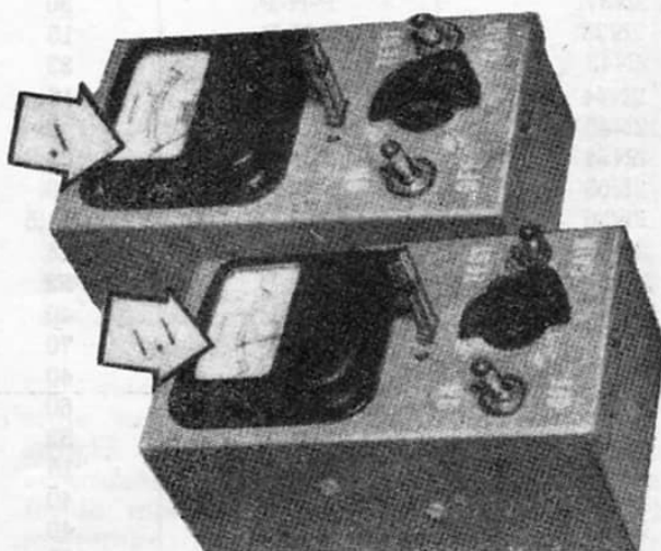
Fig. 4 - Si noti sui quadranti dei milliamperometri la variazione di deviazione degli indici, relativa alle due posizioni dell'interruttore S5.
