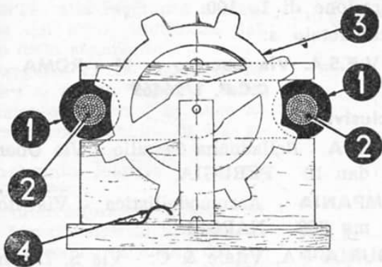
Figura 2 - Il disco rotore trovasi in posizione di partenza. Si noti infatti come una tacca risulti in contatto con la lamina a part. 4, mentre le altre si trovano sfalsate rispetto i nuclei delle elettrocalamite.
