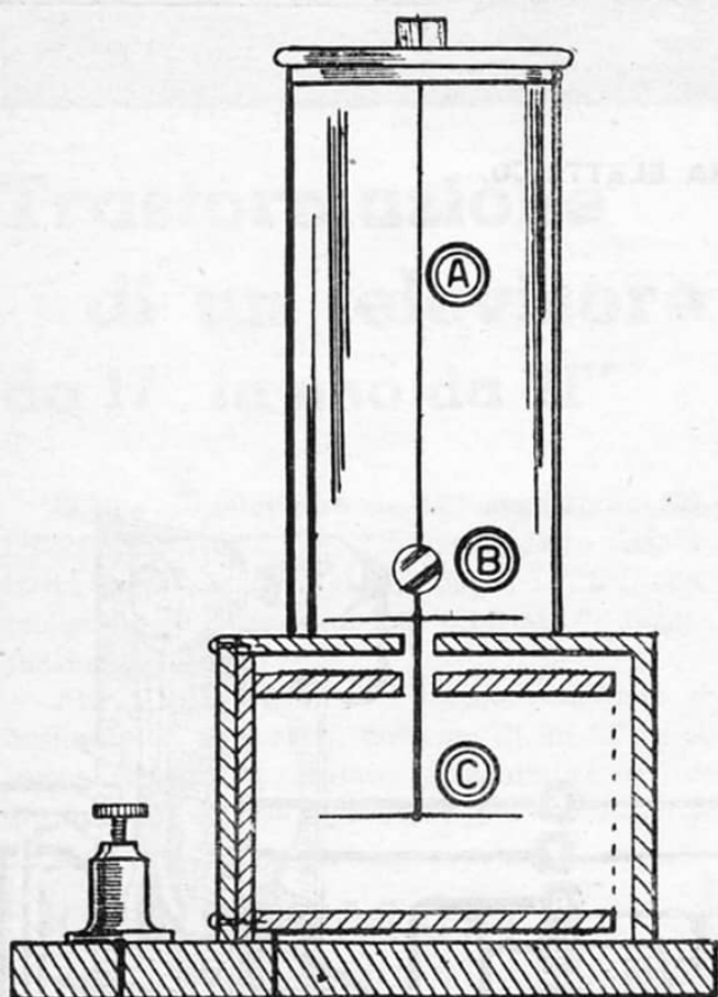
Fig. 1 - Sezione laterale dell'istrumento completato.
