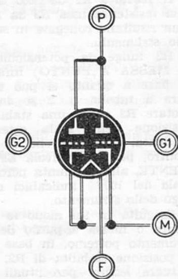
Fig. 12. — Trovandosi nella necessità di collaudare un tipo di valvola non contemplato in tabella, viene indicato in figura il modo di collegare gli elettrodi di un doppio TRIO-DO ai rispettivi terminali dell'alimentatore. Pure per detto tipo di valvola è possibile la prova separata delle due sezioni.
