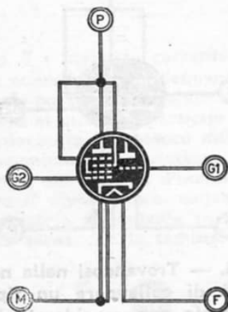
Fig. 10. — Trovandosi nella necessità di collaudare un tipo non contemplato in tabella, viene indicato a figura il modo di collegare gli elettrodi di una valvola ESO-DO-TRIO-DO o EPTODO-TRIO-DO ai rispettivi terminali dell'alimentatore. Risultando in questo tipo di valvola le due sezioni indipendenti, sarà possibile procedere al collaudo separato del triodo o dell'eptodo.
