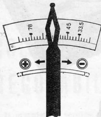
Fig. 3 - Leva laterale di messa a punto. Sulla piastrina graduata segneremo i punti corrispondenti alle velocità rilevate a mezzo dischi stroboscopici.
