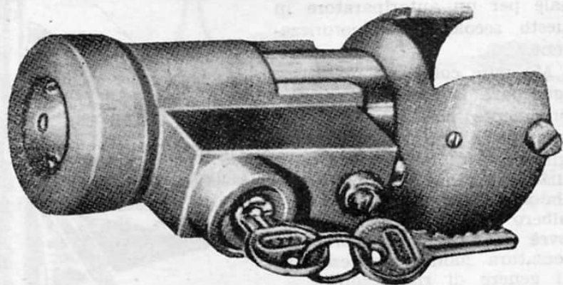
Fig. 1. — ANTIFURTO B.S.O. (bloccasterzo O.M.C.A.) con allarme acustico per FIAT 600.
