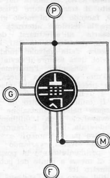
Fig. 7. — Essendo nella necessità di collaudare un tipo di valvola non contemplato in tabella, viene indicato a figura il metodo di collegamento degli elettrodi di un PENTODO ai terminali rispettivi dell'alimentatore.
