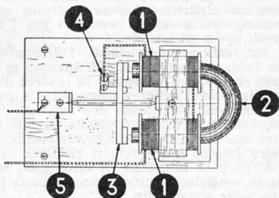
Fig. 5 - Il complesso montato visto in pianta.
