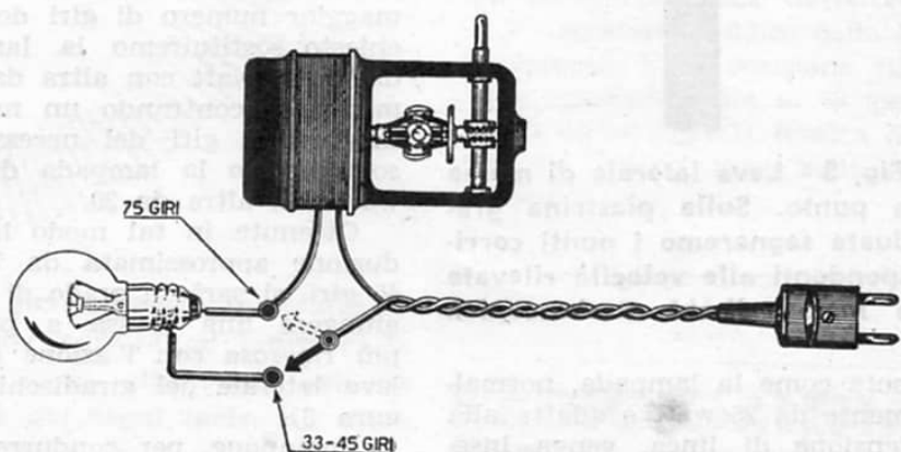
Fig. 1 - Per ridurre la velocità di un motorino da 78 a 45 giri sarà sufficiente inserire in serie al medesimo una lampada della potenza di 20-25-30 watt.
