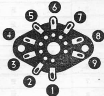
Fig. 16. — Numerazione progressiva assegnata ai piedini di uno zoccolo tipo NOVAL (vedi tabella n. 1) per l'esecuzione dei collegamenti all'alimentatore. — N. B. - Lo zoccolo s'intende visto dal disotto.
