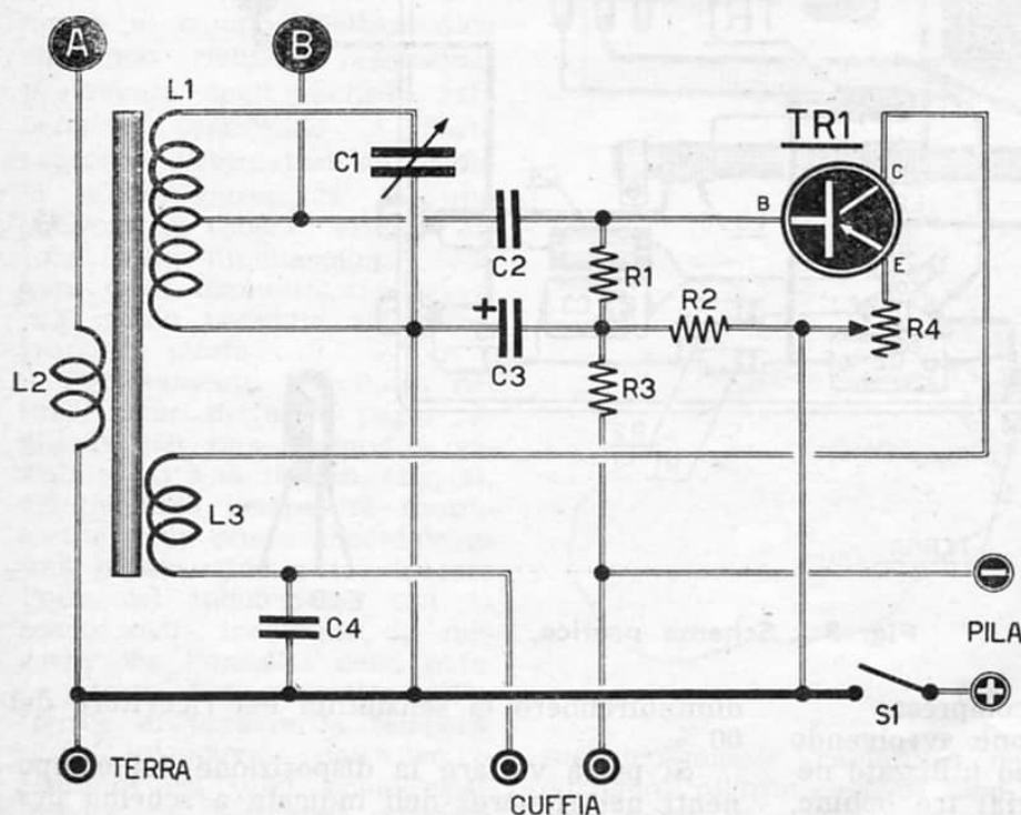
Fig. 1 - Schema elettrico.
