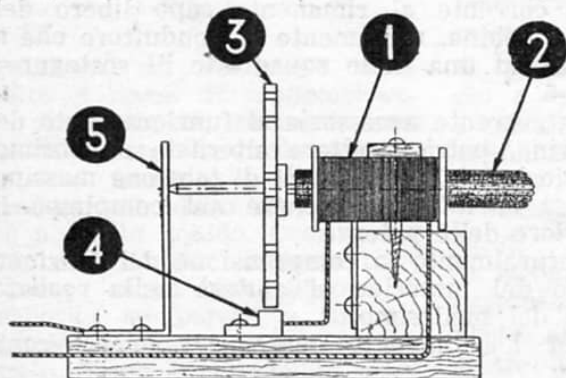
Fig. 4 - Il complesso montato visto di fianco.
