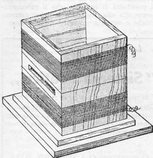
Fig. 3 - Vista prospettica del tiretto con avvolgimento realizzato.
