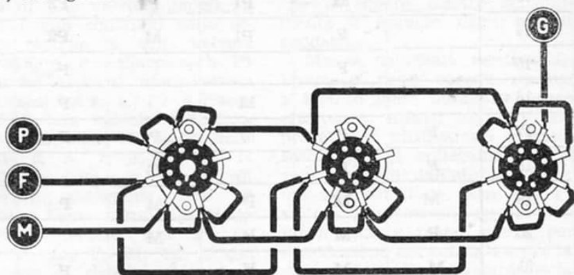
Fig. 18. — Così si presentano i collegamenti dei primi tre zoccoli (3 - 2 - 1) tipo OCTAL nel nostro provavalvole, visto, ben s'intende, dal disotto.
