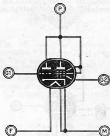
Fig. 8. — Trovandosi nella necessità di collaudare un tipo di valvola non considerato in tabella, in figura viene indicato il modo di collegare gli elettrodi di una valvola PENTODO-TRIODO ai terminali rispettivi dell'alimentatore. Come è possibile notare, del tipo di valvola considerato si possono sottoporre a collaudo le due sezioni, inserendo la griglia (G1 e G2) ai rispettivi terminali dell'alimentatore G1 e G2).
