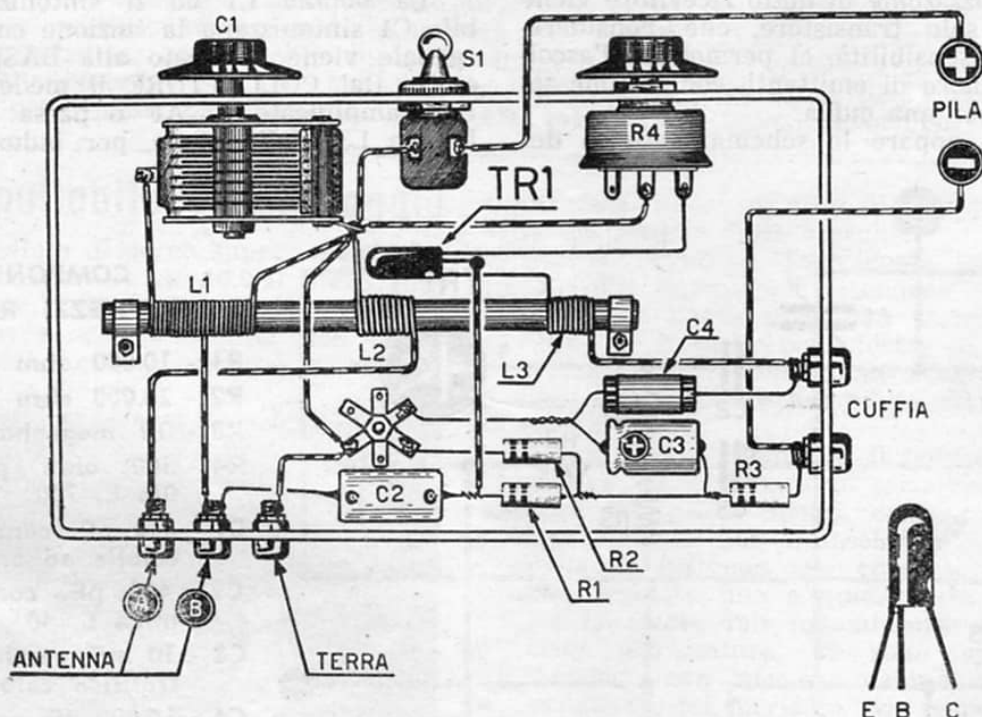
Fig. 3 - Schema pratico.
