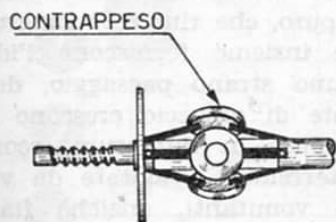
Fig. 6 - In alcuni casi sarà necessario aumentare la massa dei contrappesi del regolatore, al fine di renderlo più sensibile alle basse velocità.
