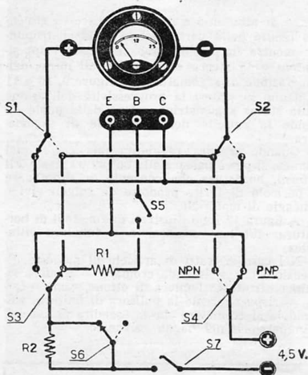
Fig. 1 - Schema elettrico del prova-transistori.
