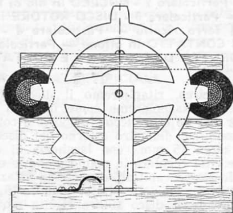
Fig. 3 - Inviando corrente nel circuito, noteremo come le tacche vengano attratte dalle espansioni polari delle elettrocalamite, dando così inizio al ciclo di rotazione del disco rotore. Evidentemente il distacco della tacca dalla lamina determinerà la cessazione del passaggio di corrente; ma la forza d'inerzia, di cui risulterà dotato il disco rotore, consentirà l'ottavo di giro necessario all'entrata in contatto della successiva tacca con la lamina.
