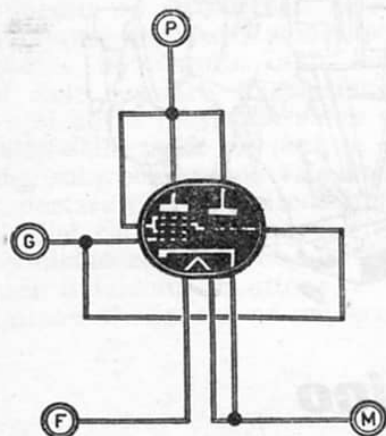
Fig. 9. — Essendo nella necessità di sottoporre a collaudo un tipo di valvola non contemplato in tabella, viene indicato a figura il metodo di collegamento degli elettrodi di una valvola convertitrice EP-TODO o PENTAGRIGLIA ai terminali rispettivi dell'alimentatore.
