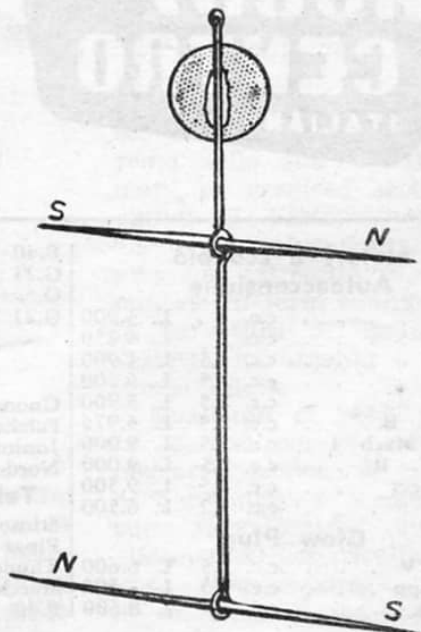
Fig. 4 - Complesso aghi magnetizzati. Si noti l'inversione delle polarità degli aghi stessi.
