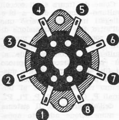
Fig. 13. — Numerazione progressiva assegnata ai piedini di uno zoccolo tipo OCTAL (vedi tabella n. 1) per l'esecuzione dei collegamenti all'alimentatore. — N. B. Lo zoccolo s'intende visto dal disotto.
