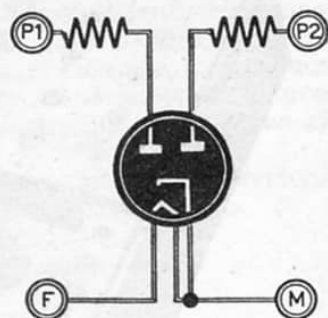
Fig. 11. — Essendo nella necessità di sottoporre a collaudo un tipo di valvola non contemplato in tabella, viene indicato a figura il metodo di collegamento degli elettrodi di una valvola raddrizzatrice ai rispettivi terminali dell'alimentatore. Si noti come, in serie alle due sezioni delle placche, risultino inserite due resistenze, il cui valore dovrà essere ricercato sperimentalmente ad impedire che la lancetta dello strumento si porti a fondo scala.
