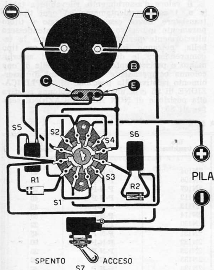
Fig. 2 - Schema pratico del prova-transistori.
