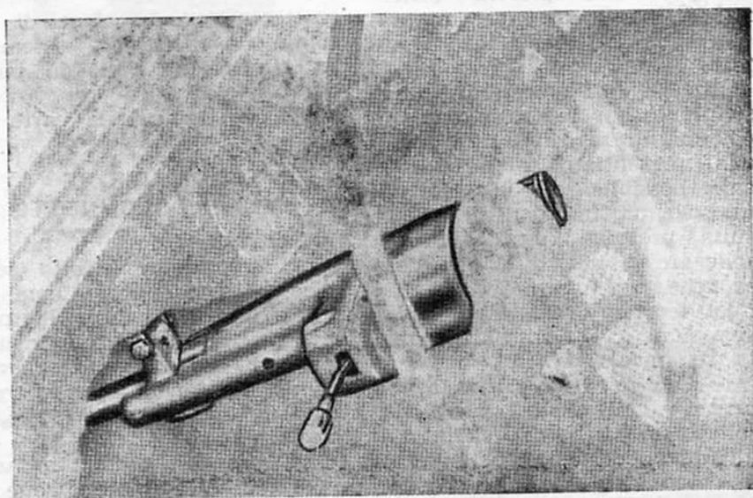
Fig. 2. — BRANC-COBO gruppo unificato antifurto cambioluce per FIAT 600.
