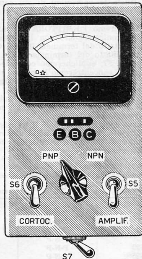
Fig. 3 - Pannello frontale del prova-transistori.
