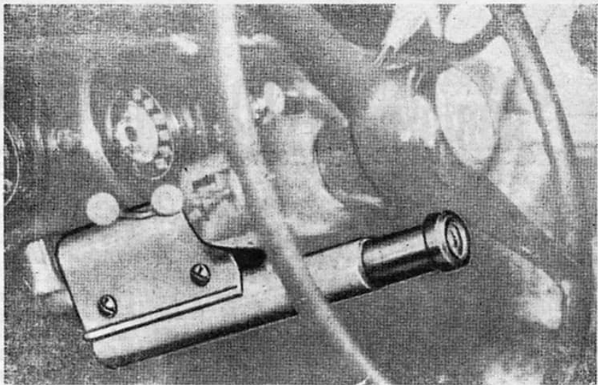
Fig. 3. — BRANC antifurto fermasterzo con allarme acustico per tutti i modelli di vetture FIAT.
