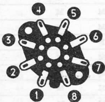
Fig. 14. — Numerazione progressiva assegnata ai piedini di uno zoccolo tipo RIMLOK (vedi tabella n. 1) per l'esecuzione dei collegamenti all'alimentatore. — N. B. - Lo zoccolo s'intende visto dal disotto.
