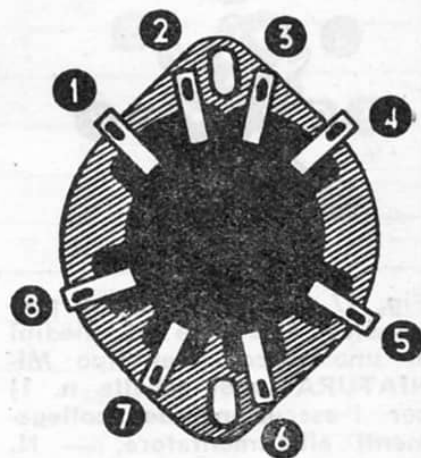
Fig. 15. — Numerazione progressiva assegnata ai piedini di uno zoccolo del tipo a VA-SCHETTA (vedi tabella n. 1) per l'esecuzione dei collegamenti all'alimentatore. — N. B. - Lo zoccolo s'intende visto dal disotto.
