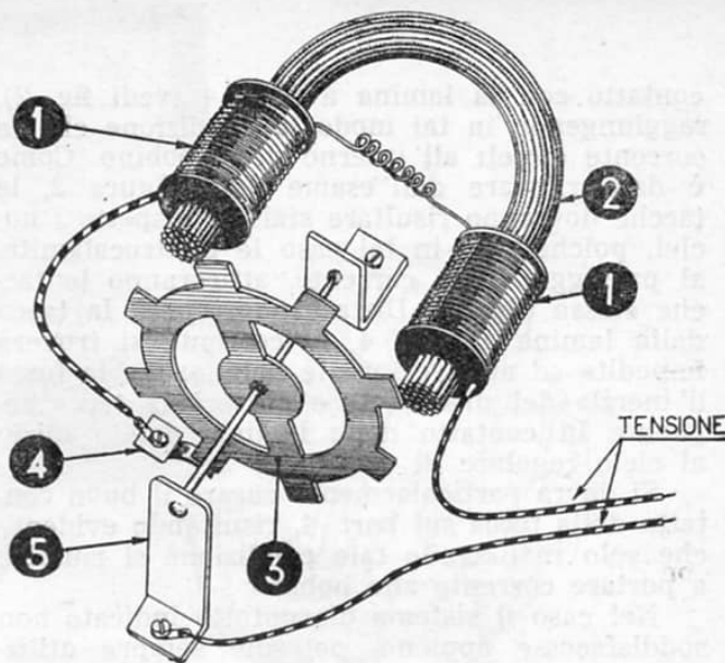
Fig. 1 - Vista prospettica del complesso scomposto nei componenti. — Particolare 1 - BOBINE — Particolare 2 - NUCLEO in filo di ferro ricotto — Particolare 3 - DISCO ROTORE in lamiera di ferro ricotto — Particolare 4 - LAMINA DI CONTATTO in ottone — Particolare 5 - SQUADRETTA DI SOSTEGNO E CONTATTO.
