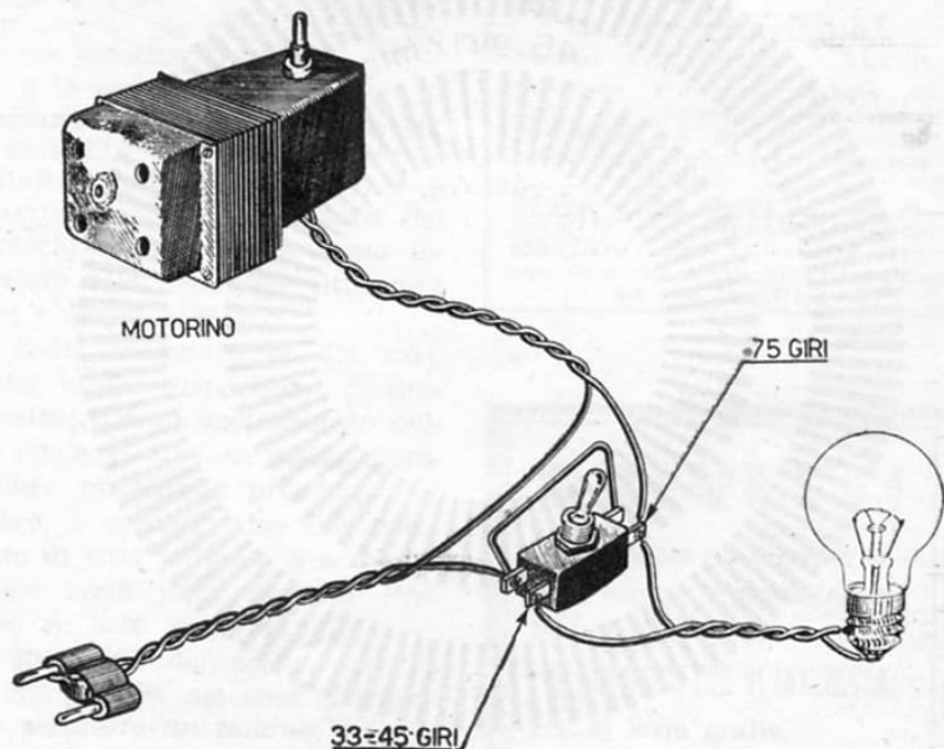
Fig. 2 - Schema pratico dell'applicazione. Per l'inserimento o il disinserimento della lampada si è ricorsi all'ausilio di un deviatore a levetta.
