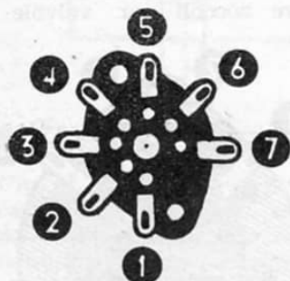
Fig. 17. — Numerazione progressiva assegnata ai piedini di uno zoccolo del tipo MINIATURA (vedi tabella n. 1) per l'esecuzione dei collegamenti all'alimentatore. — N. B. - Lo zoccolo s'intende visto dal disotto
