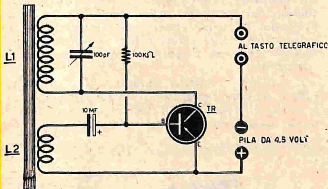
Fig. 1 - Schema elettrico.
