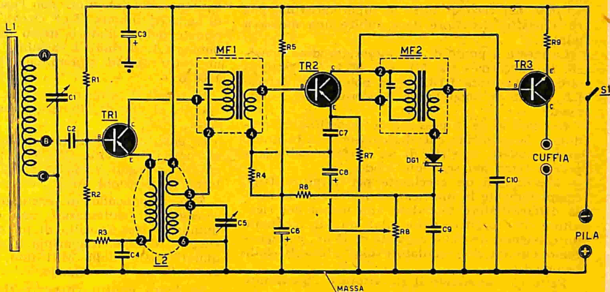
Fig. 1 - Schema elettrico
