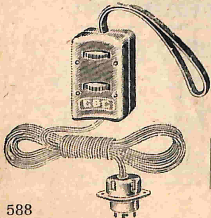
Fig. 1 - Telecomando della GBC tipo M/597/2 completo di cordone e spina a quattro terminali per il collegamento al televisore.
