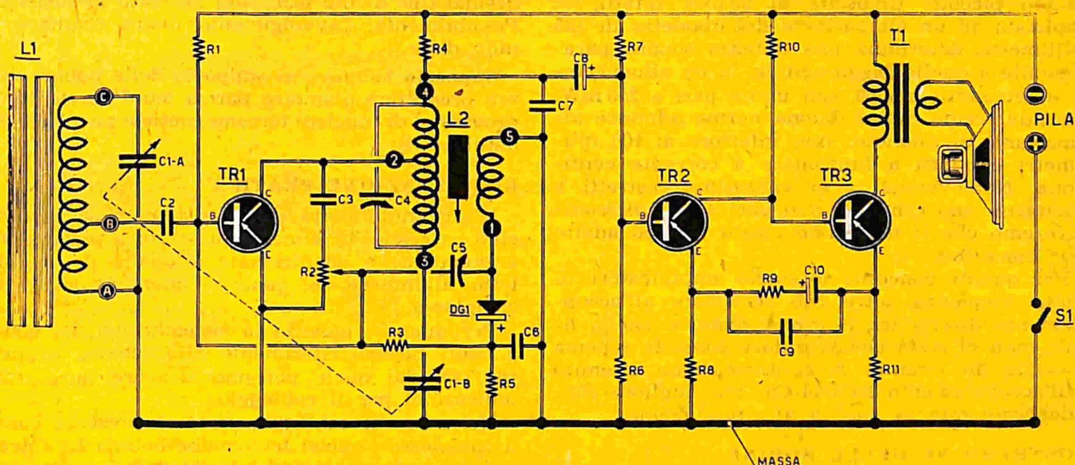
Fig. 1 - Schema elettrico.
