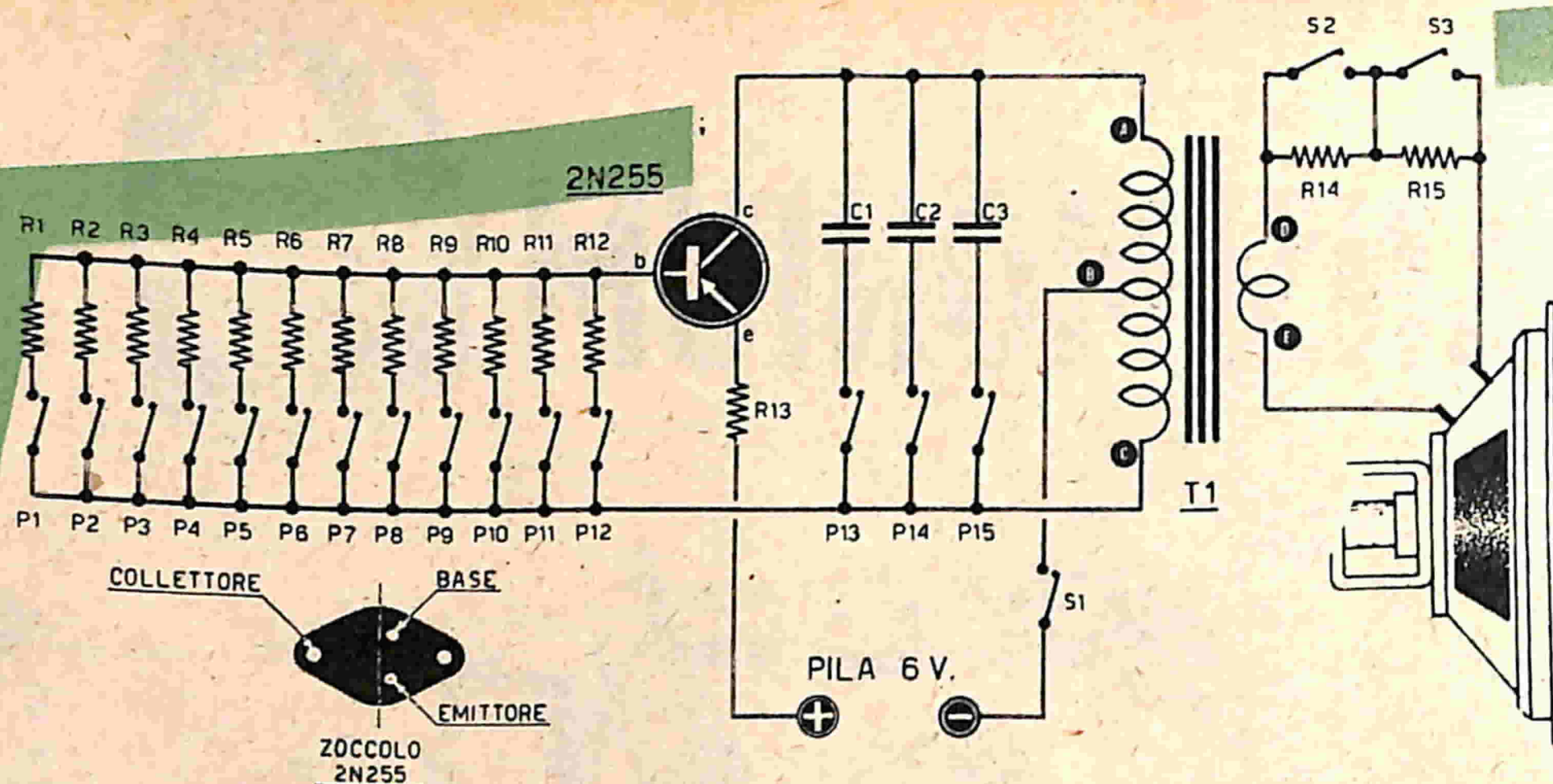
Fig. 1 - Schema elettrico.
