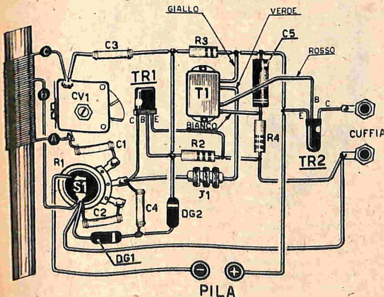
Figura 2 - Schema pratico
