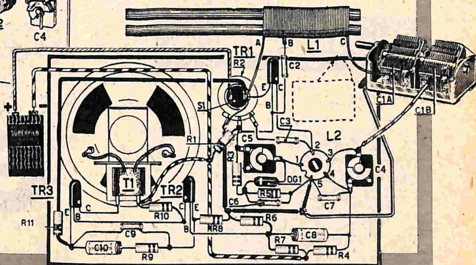
Fig. 4 - Schema pratico.
