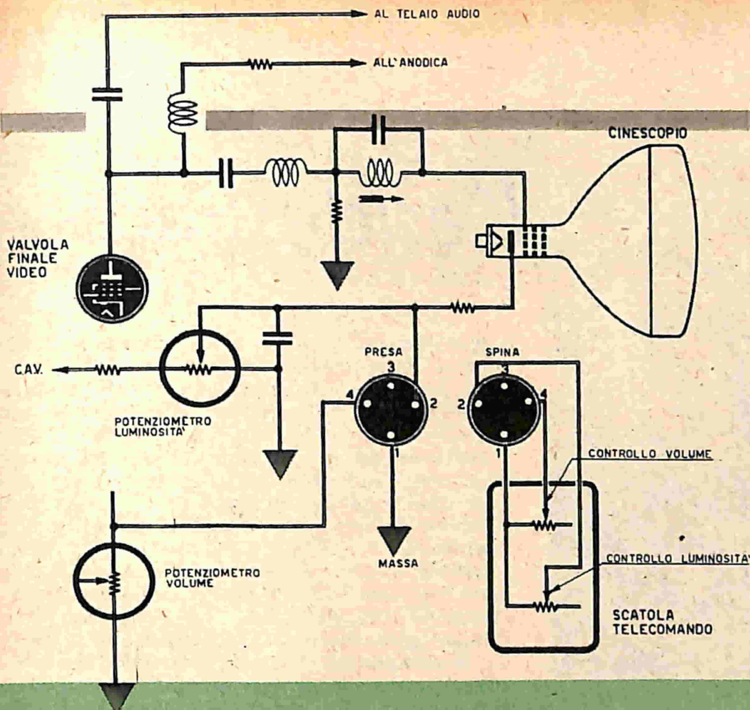
Fig. 2 - Sistema di collegamento del telecomando in un televisore il cui segnale video risulti applicato alla griglia del tubo cinescopio.
