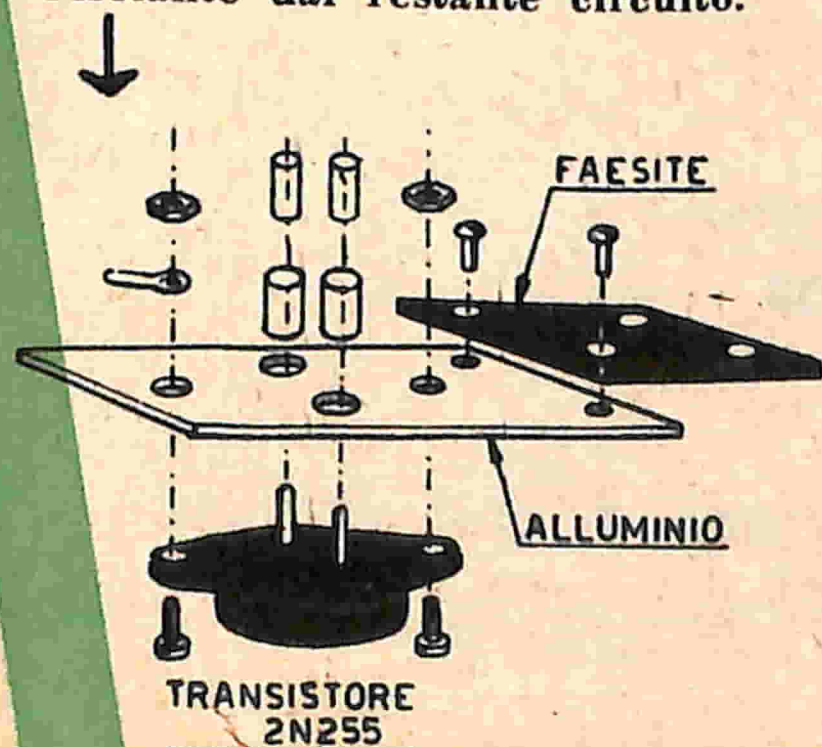
Fig. 4 - Lo zoccolo del transistor di potenza 2N255 viene montato su piastra d'alluminio, la quale a sua volta viene sistemata su faesite per l'isolante dal restante circuito.
