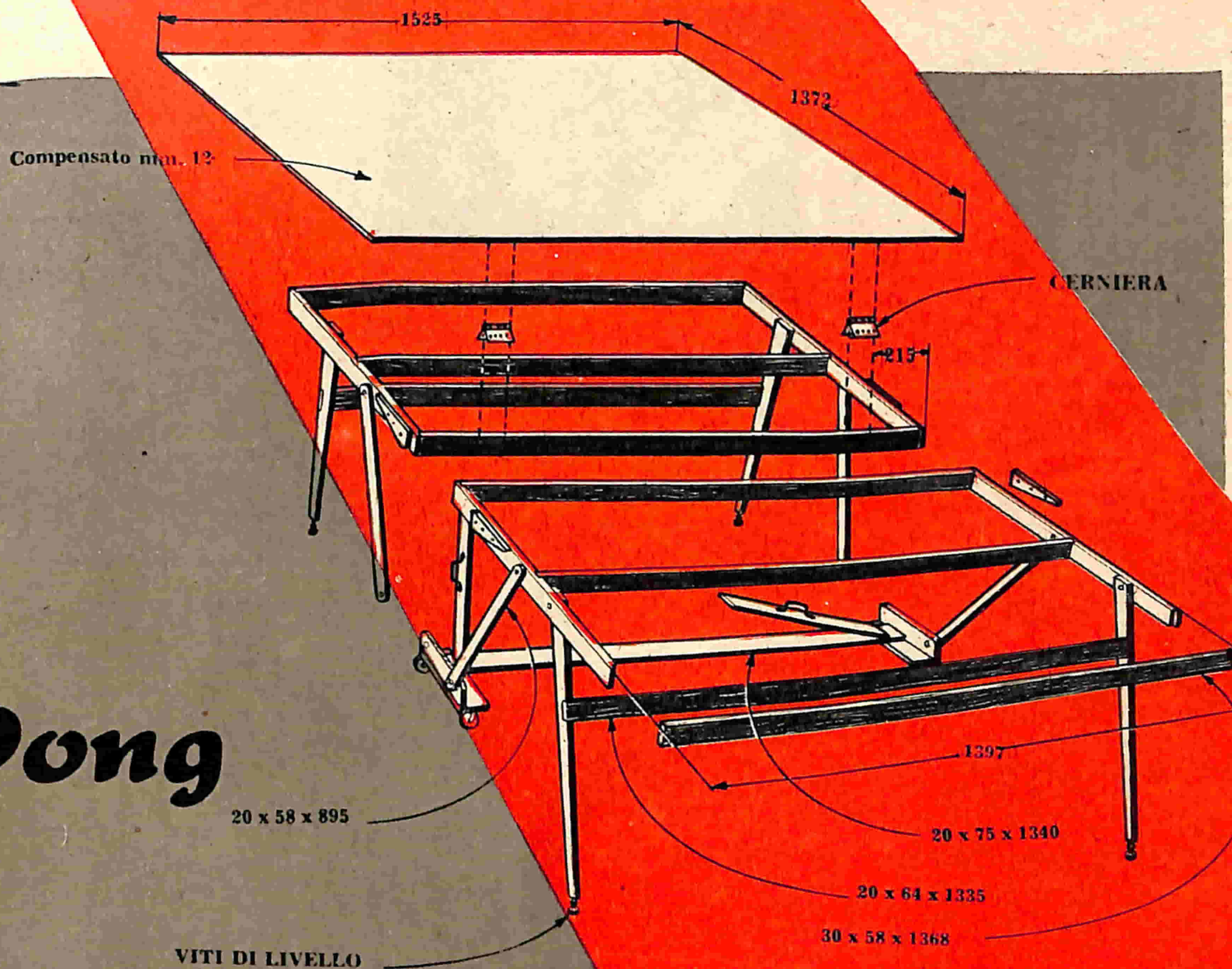
Fig. 1 - Dimensioni elementi componenti il tavolo.
