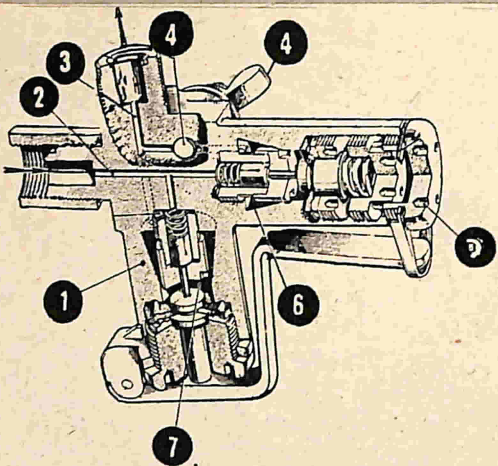
Fig. 6 - Alla valvola BY-PASS è affidato il compito di regolare l'afflusso dell'ossigeno al sacco polmone a pressione desiderata. La valvola BY-PASS viene pure utilizzata dai subacquei quale dispositivo di sicurezza. Infatti — avvertendo sintomi di malessere — si agirà sul BY-PASS, il quale — richiamando maggior quantità di ossigeno nel sacco polmone — gonfierà il medesimo e il subacqueo sarà riportato a superficie. A figura la valvola BY-PASS sezionata: 1) involucro metallico della valvola; 2) condotti ad alta pressione che si collegano alla bombola; 3) condotti a bassa pressione che si collegano al sacco polmone; 4) manopola dell'erogatore; 5) fori per chiave a tubo; 6) riduttore di pressione; 7) comando del flusso.
