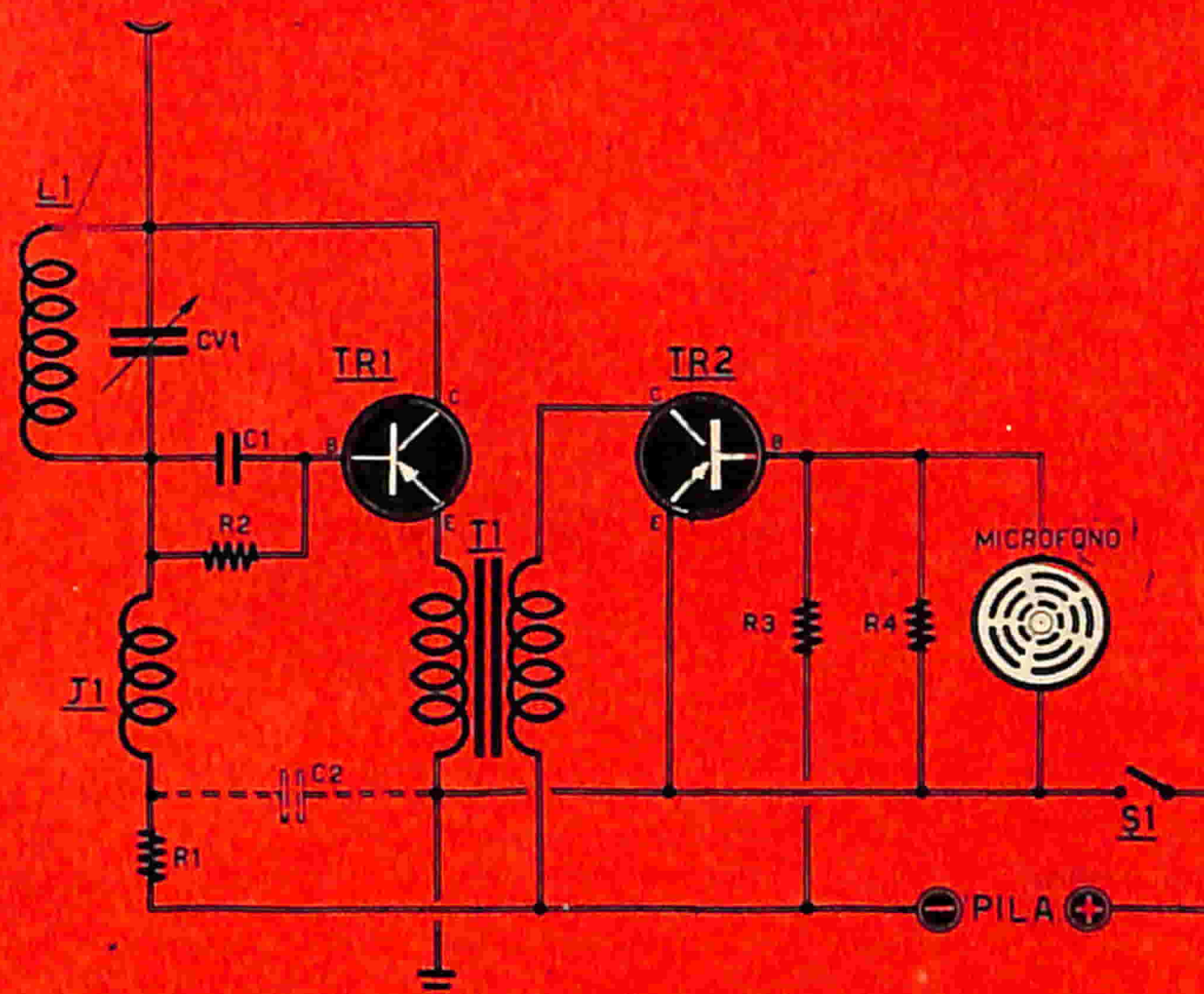
Fig. 1 - Schema elettrico.
