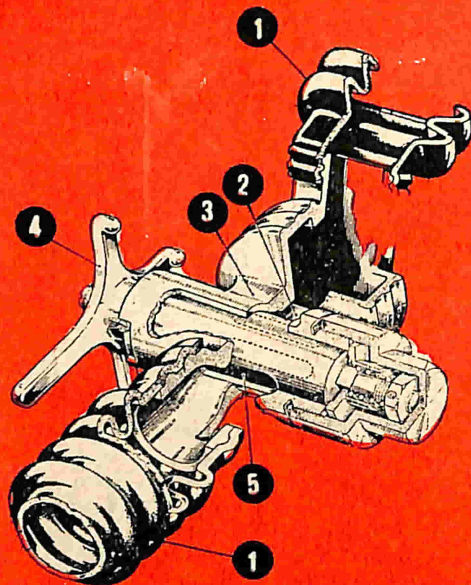
Fig. 3 - Al rubinetto a 3 vie è affidato il compito di comandare il passaggio dalla respirazione atmosferica a quella ad ossigeno. Aprendo il condotto dell'ossigeno contenuto nel sacco polmone viene a chiudersi automaticamente il condotto dell'aria atmosferica e viceversa.
