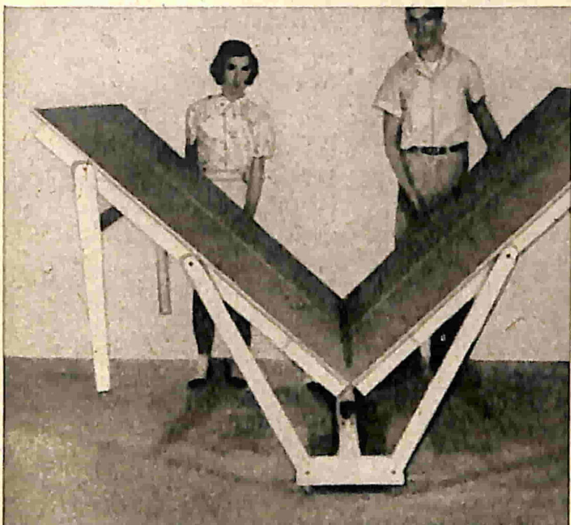
Fig. 8 - Fase di apertura del tavolo.
