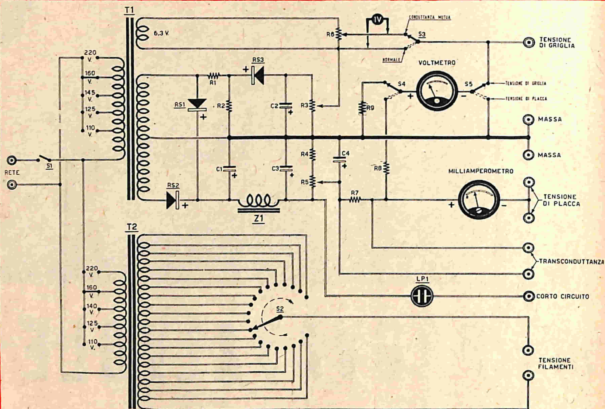
Fig. 1 - Schema elettrico.
