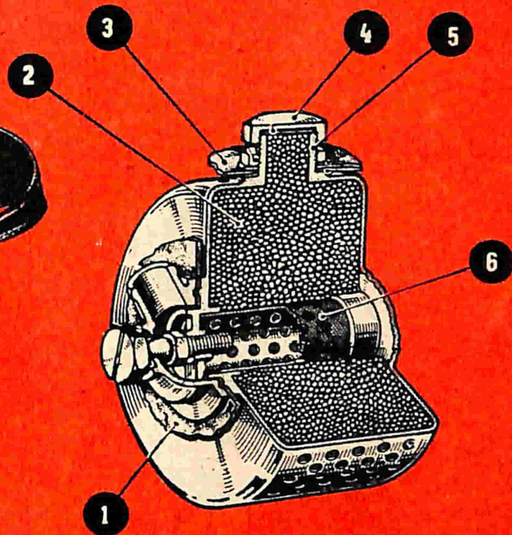
Fig. 5 - Filtro o cartuccia epuratrice a calce sodata. La calce da utilizzare per il riempimento della cartuccia deve essere asciutta, di colore bianco, sufficientemente dura sì da risultare difficile il ridurla in polvere con le dita. Prima di venire introdotta all'interno della cartuccia, la calce verrà passata attraverso un setaccio fine, allo scopo di eliminare i granuli troppo grossi.
