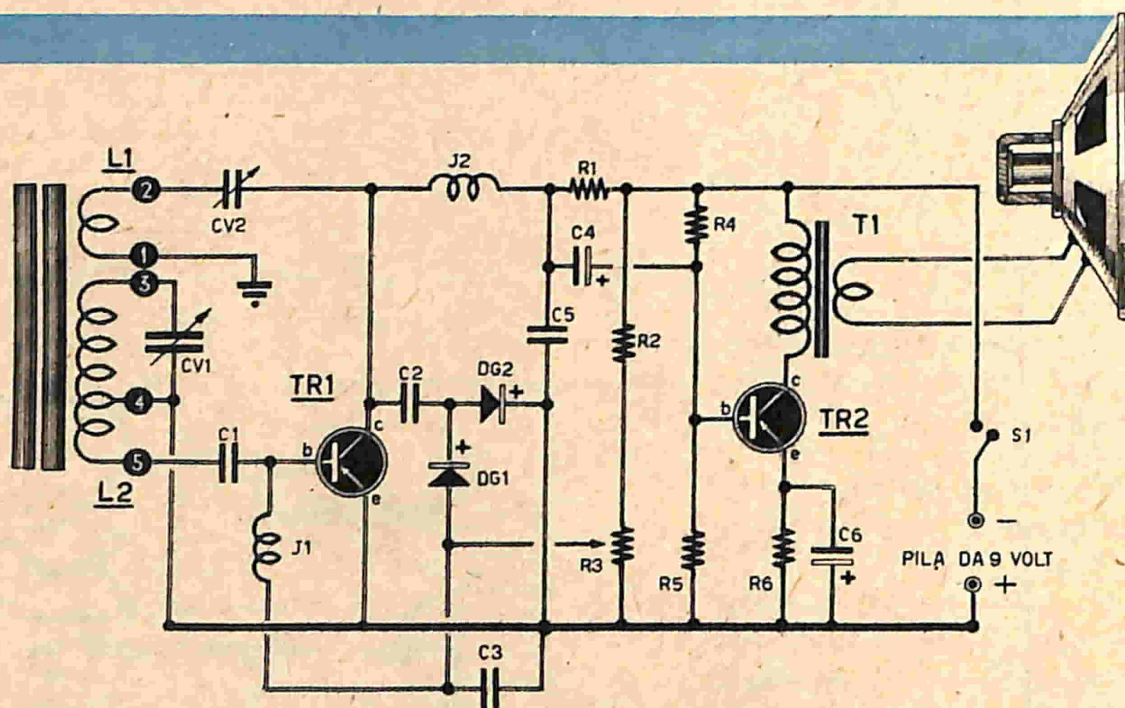
Fig. 1 - Schema elettrico.
