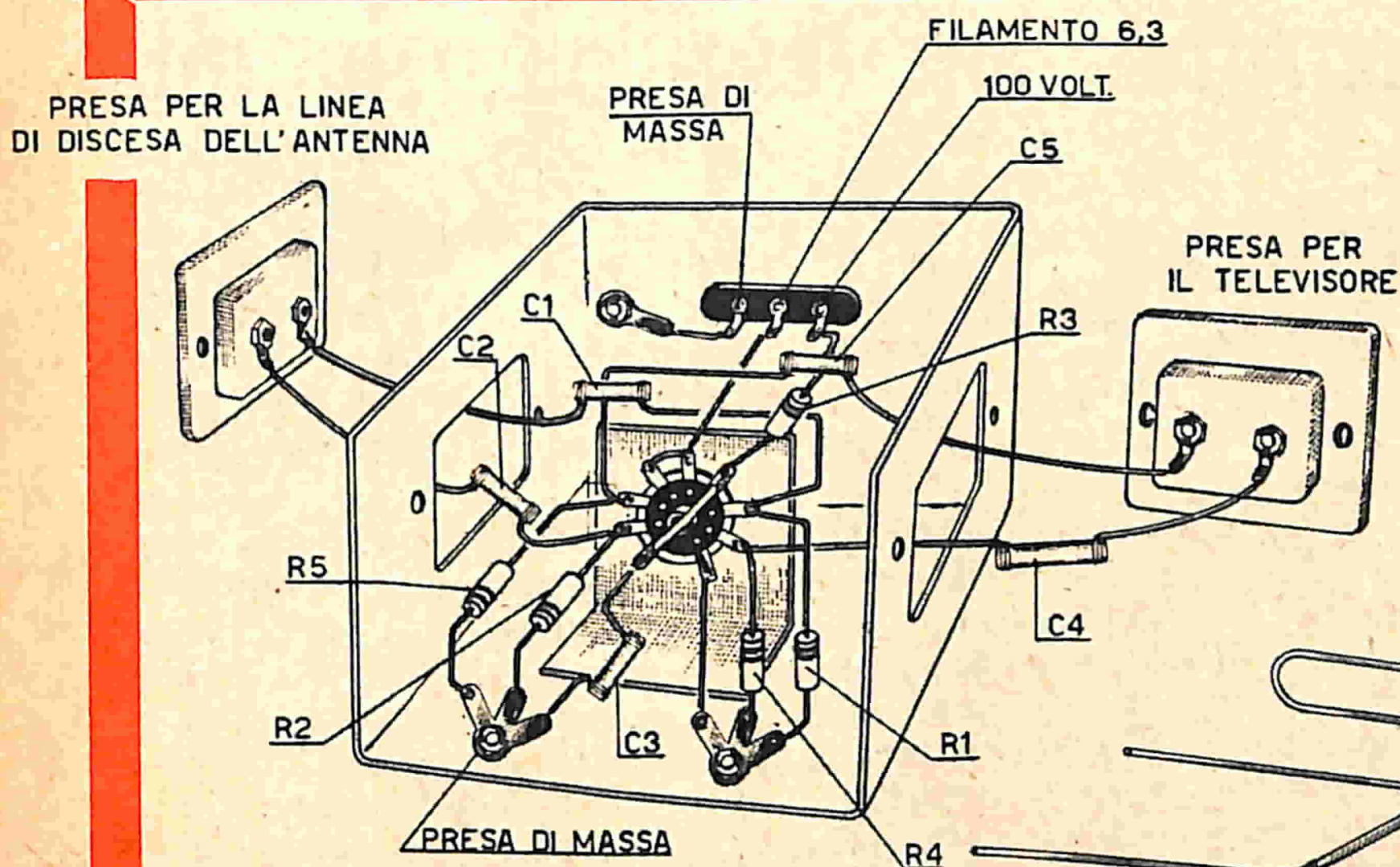
Fig. 2 - Schema pratico.
