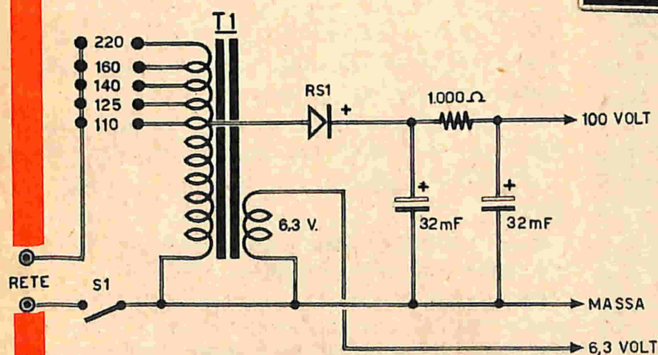
Fig. 3 - Alimentatore separato.
