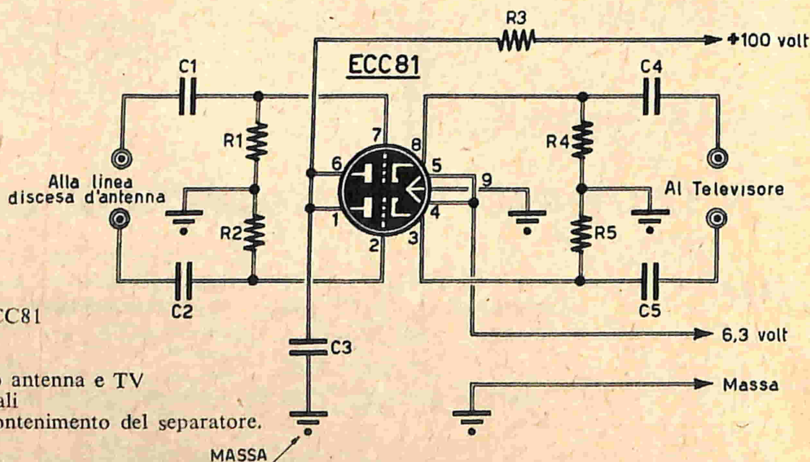
Fig. 1 - Schema elettrico.
