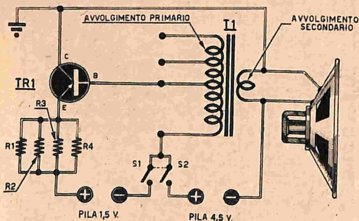
Fig. 1 - Schema elettrico.
