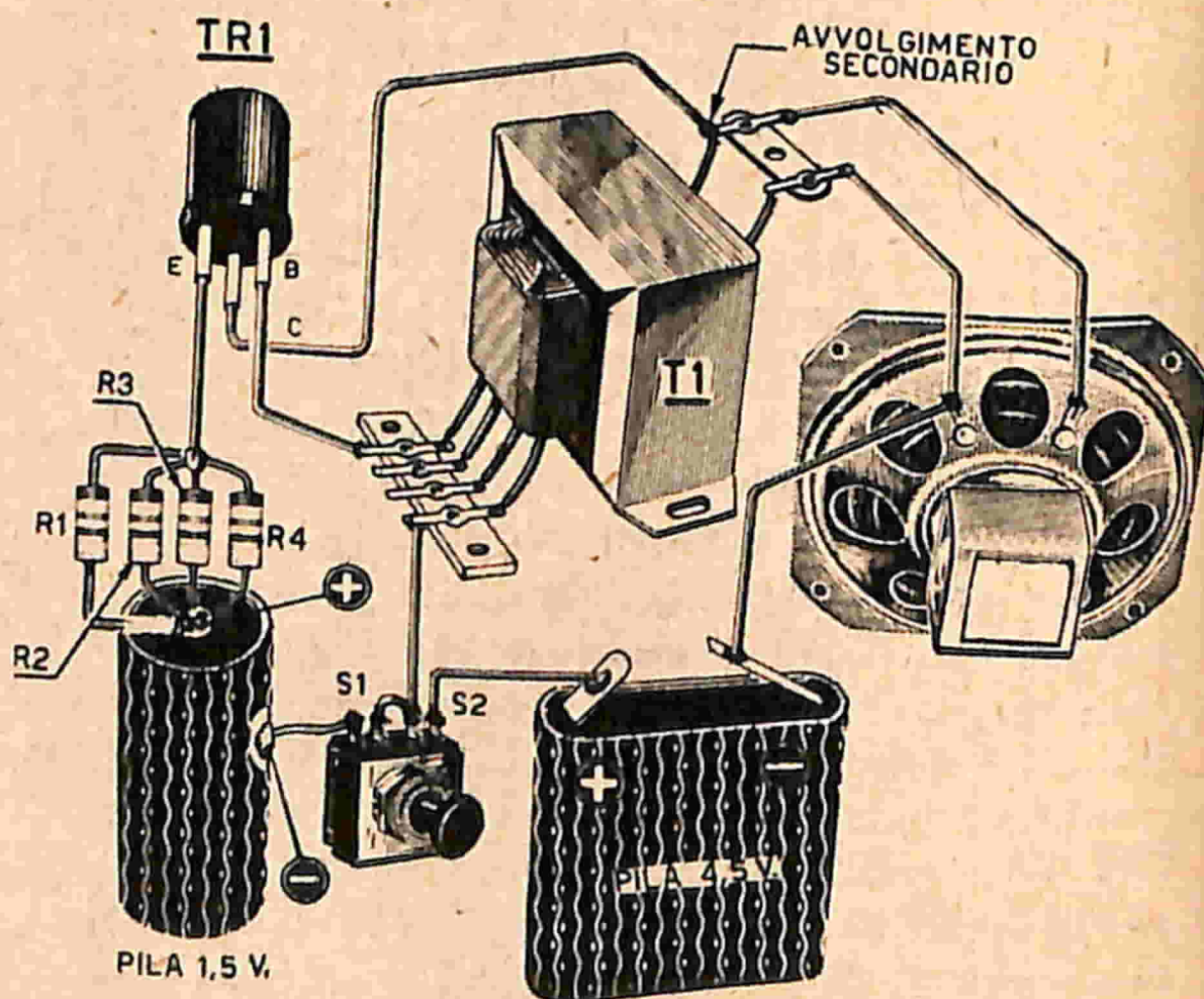
Fig. 2 - Schema pratico.
