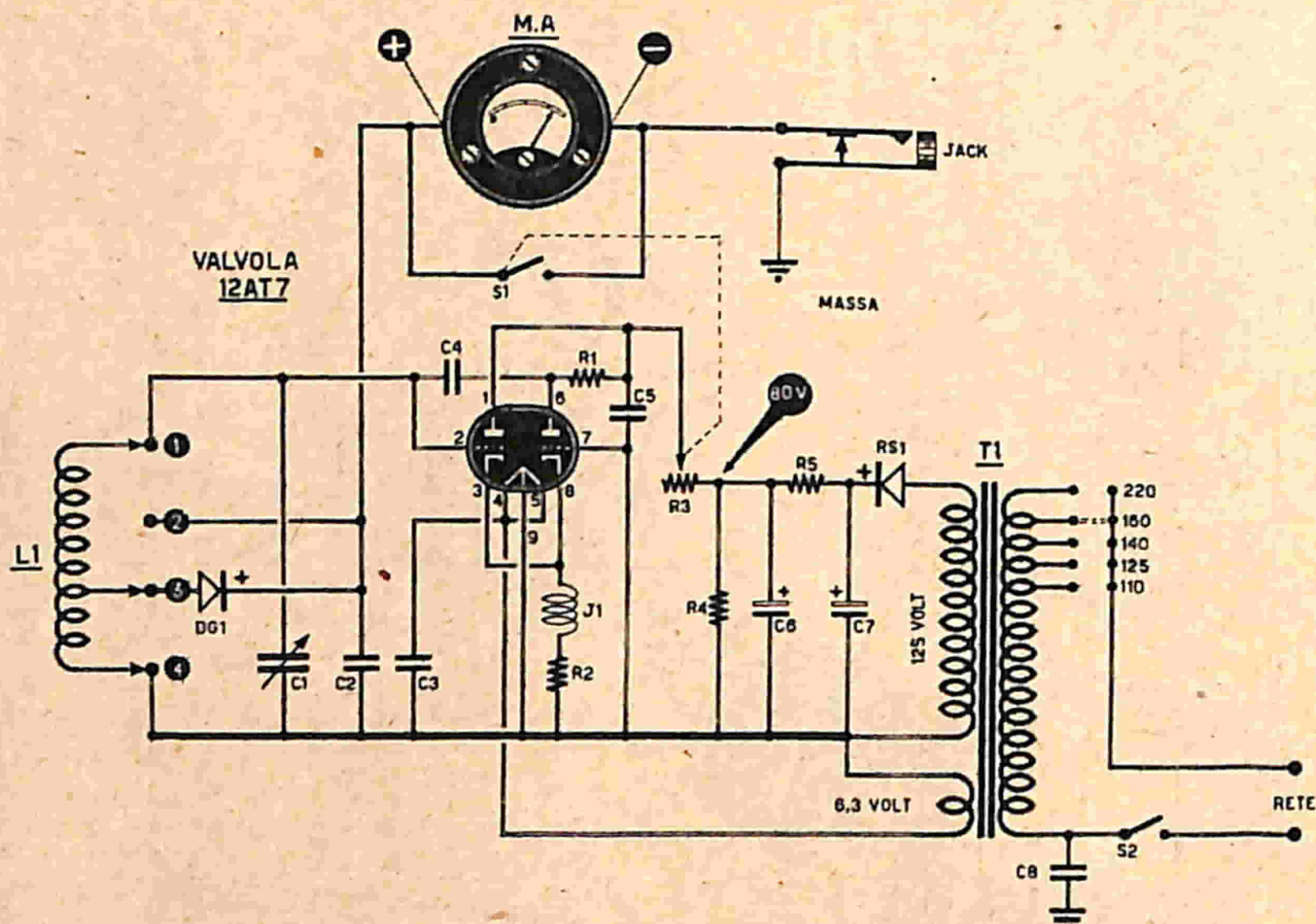
Fig. 1 - Schema elettrico ELENCO COMPONENTI E PREZZI RELATIVI
