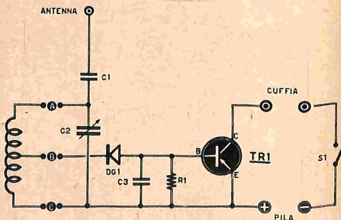
Fig. 1 - Schema elettrico
