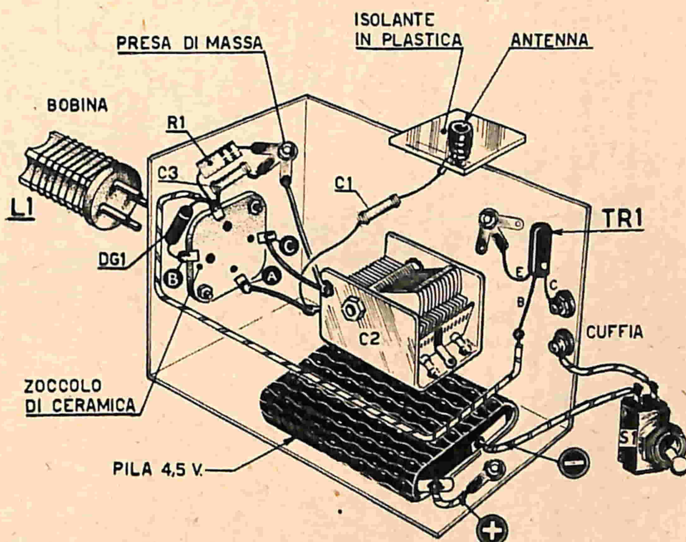
Fig. 2 - Schema pratico
