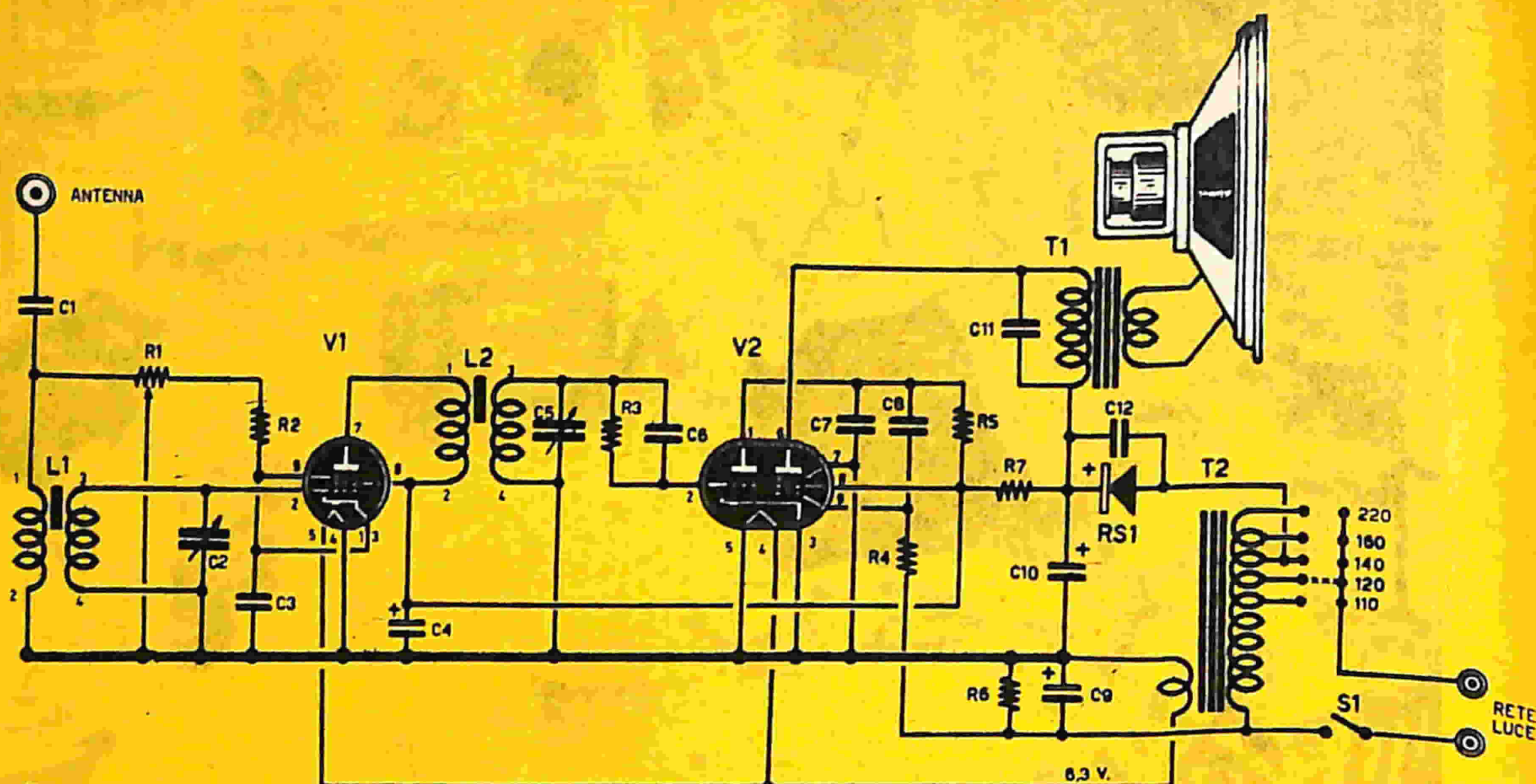
Fig. 1 SCHEMA ELETTRICO COMPONENTI
