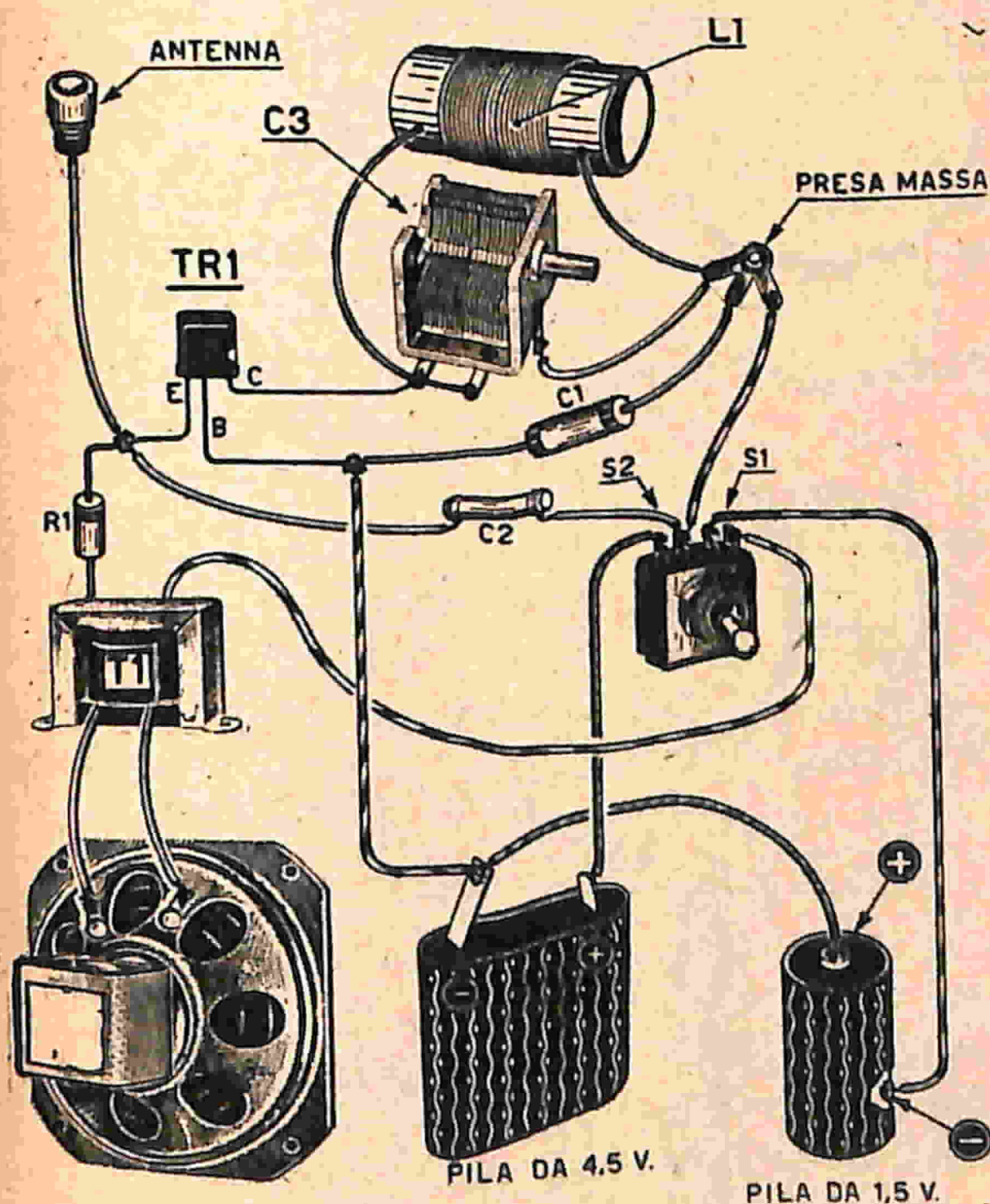
Fig. 2 - Schema pratico
