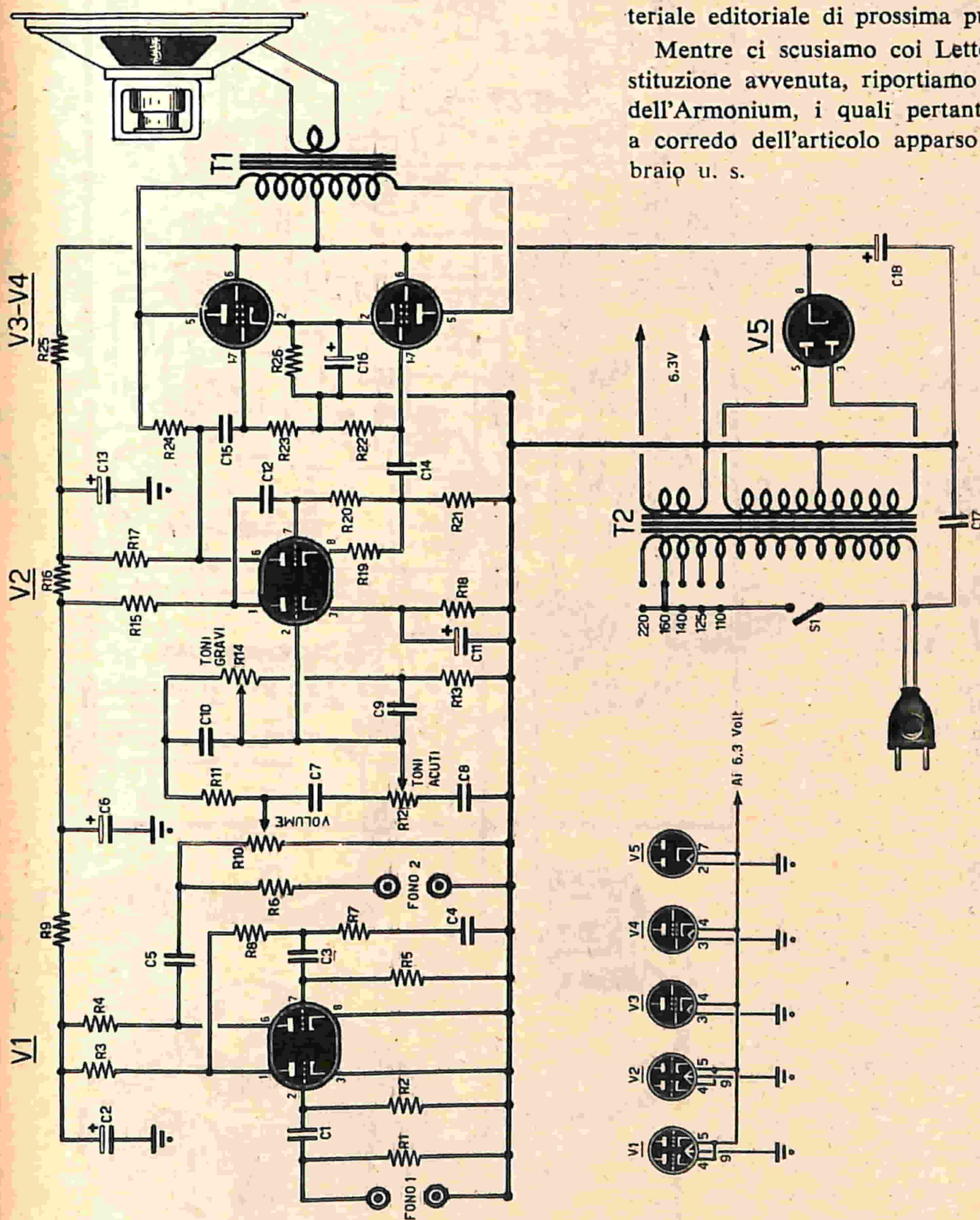
Fig. 1 - Schema elettrico
