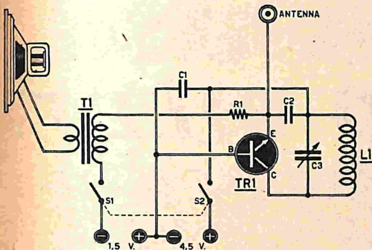
Fig. 1 - Schema elettrico.
