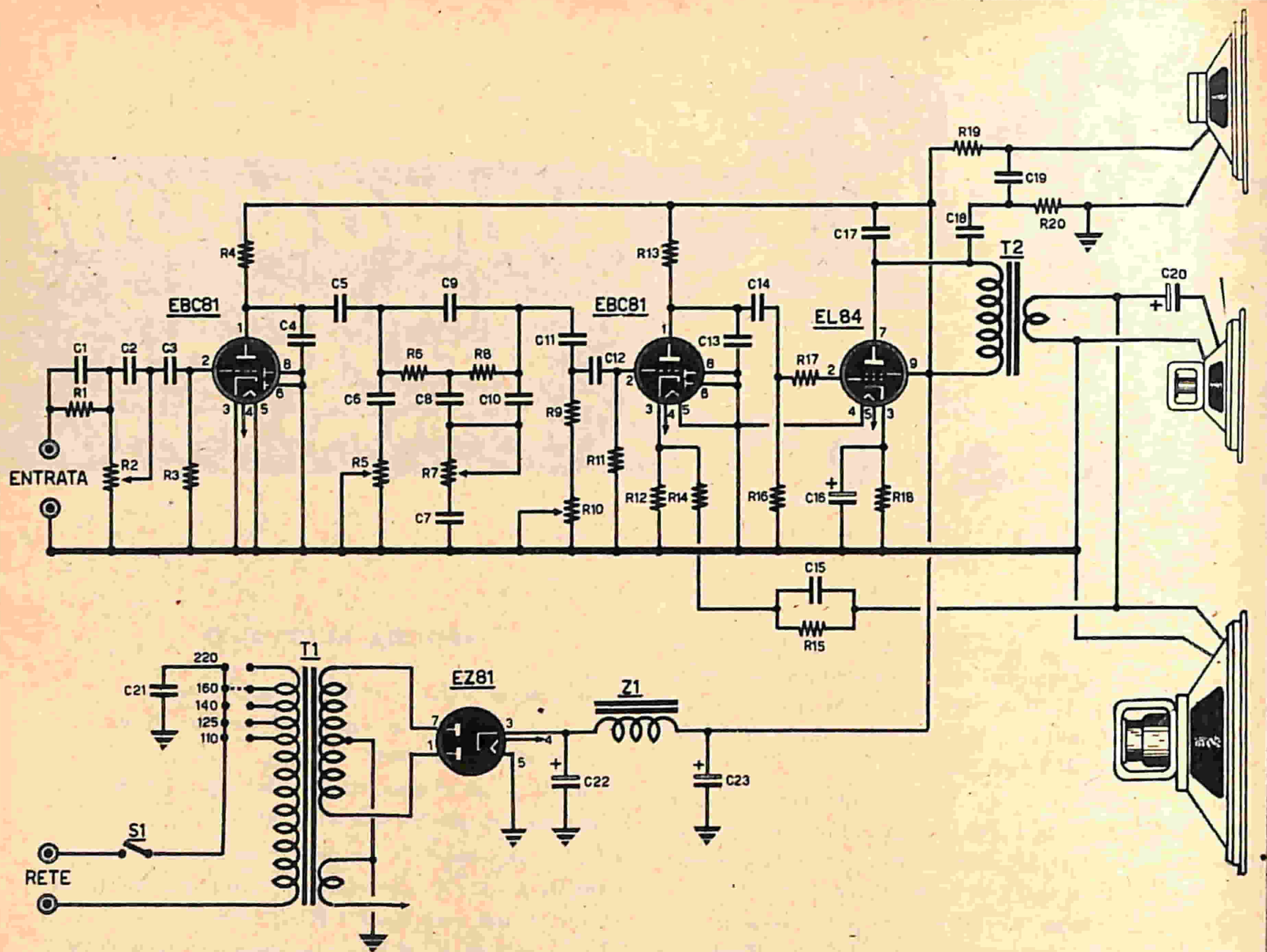
Fig. 1 - Schema elettrico.
