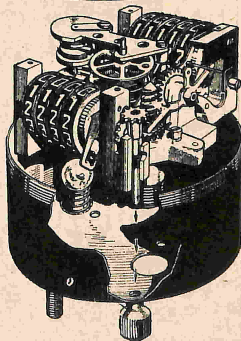
Fig.4 - Il tachimetro a lancetta è il tipo più comune. Il disco di alluminio indotto è direttamente collegato alla lancetta. In figura il tachimetro smontato completo di contachilometri ed il tipo semplificato.
