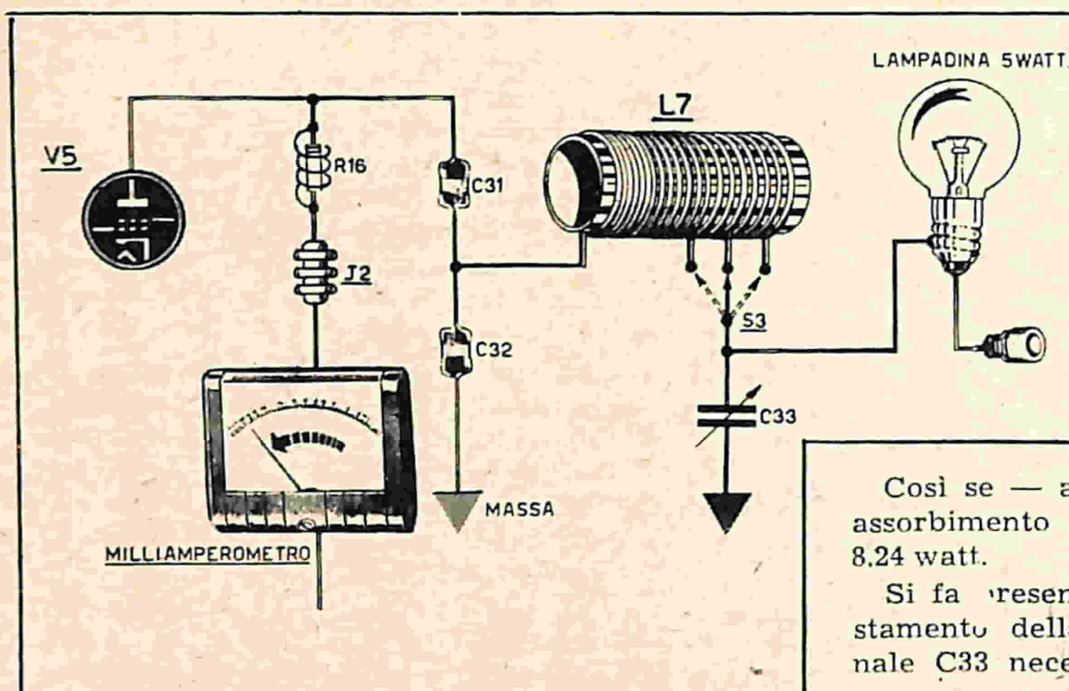
Fig. 16 - Portata a termine la taratura dello stadio finale, necessiterà sintonizzare l'antenna. Allo scopo inseriremo — in serie alla presa d'antenna — una lampada da 5 watt. L'assorbimento indicato dallo strumento dovrà risultare pari a quello di cui a figura 15.
