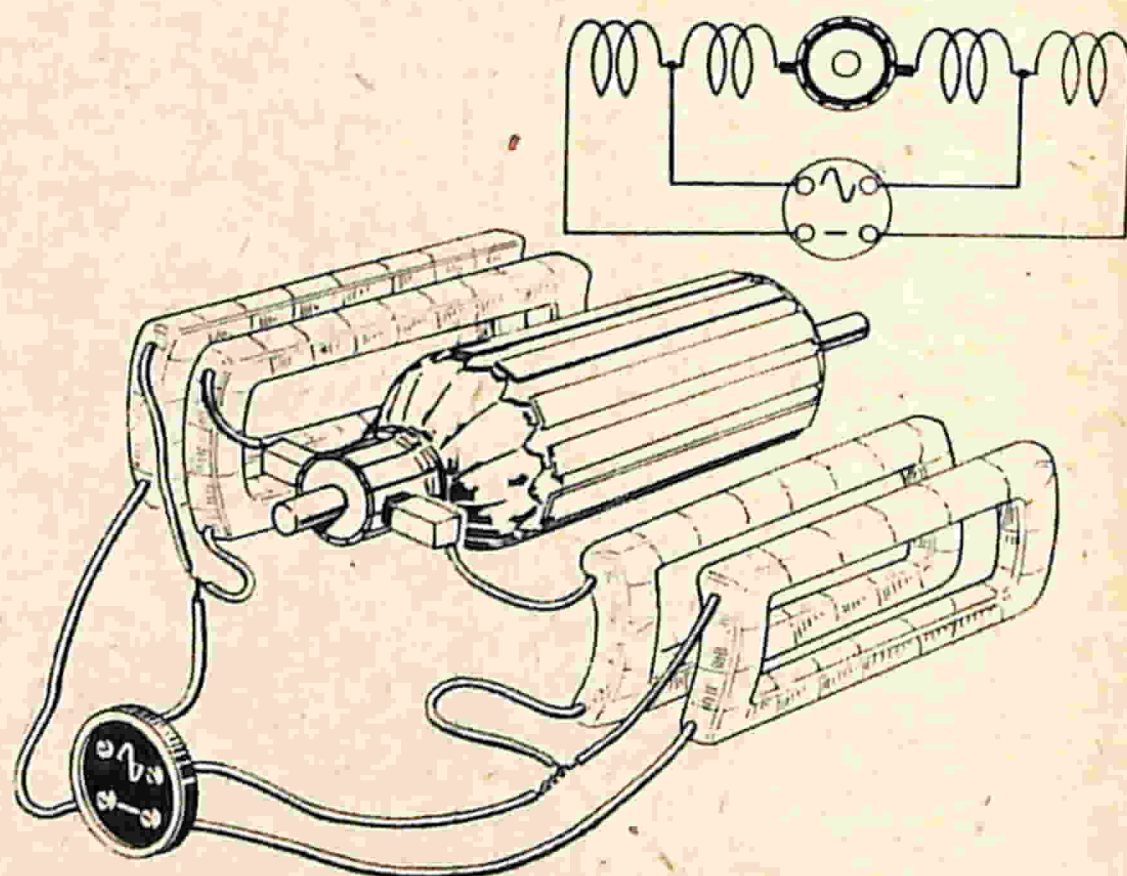
Fig.1 - Alimentando il motorino ai morsetti segnati con ~ il medesimo funziona in alternata; dando invece corrente ai morsetti — esso funziona con corrente continua.
