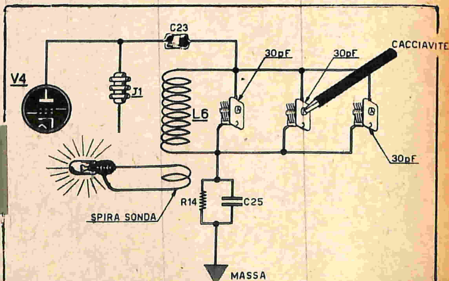
Fig. 13 - Non disponendo di una lampada al neon, ci serviremo di una lampada da 6,3 volt che preveda l'accoppiamento a due spire.
