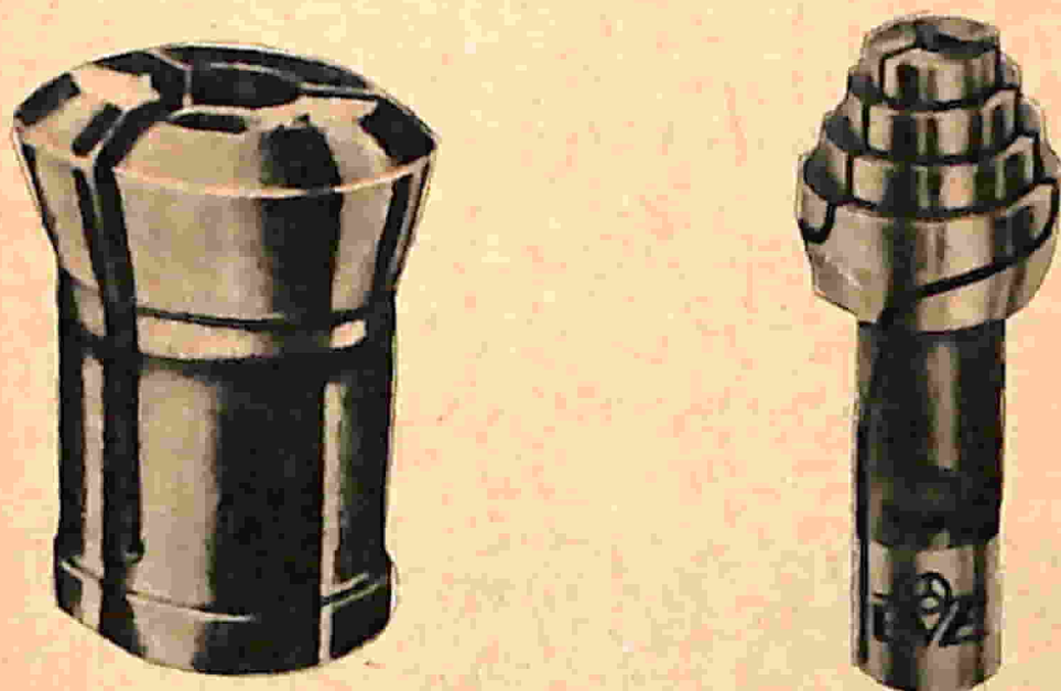
Fig. 1 - Tipo di pinza espansibile che si adatta a tutte le macchine che portano pinze con chiusura a trazione e chiusura a spinta. Trattasi di pinze temperate e a ganasce semidure, sì che sia possibile l'adattamento ai profili dei pezzi in lavorazione. Fig. 2 - Altro tipo di pinze espansibili in acciaio temperato.
