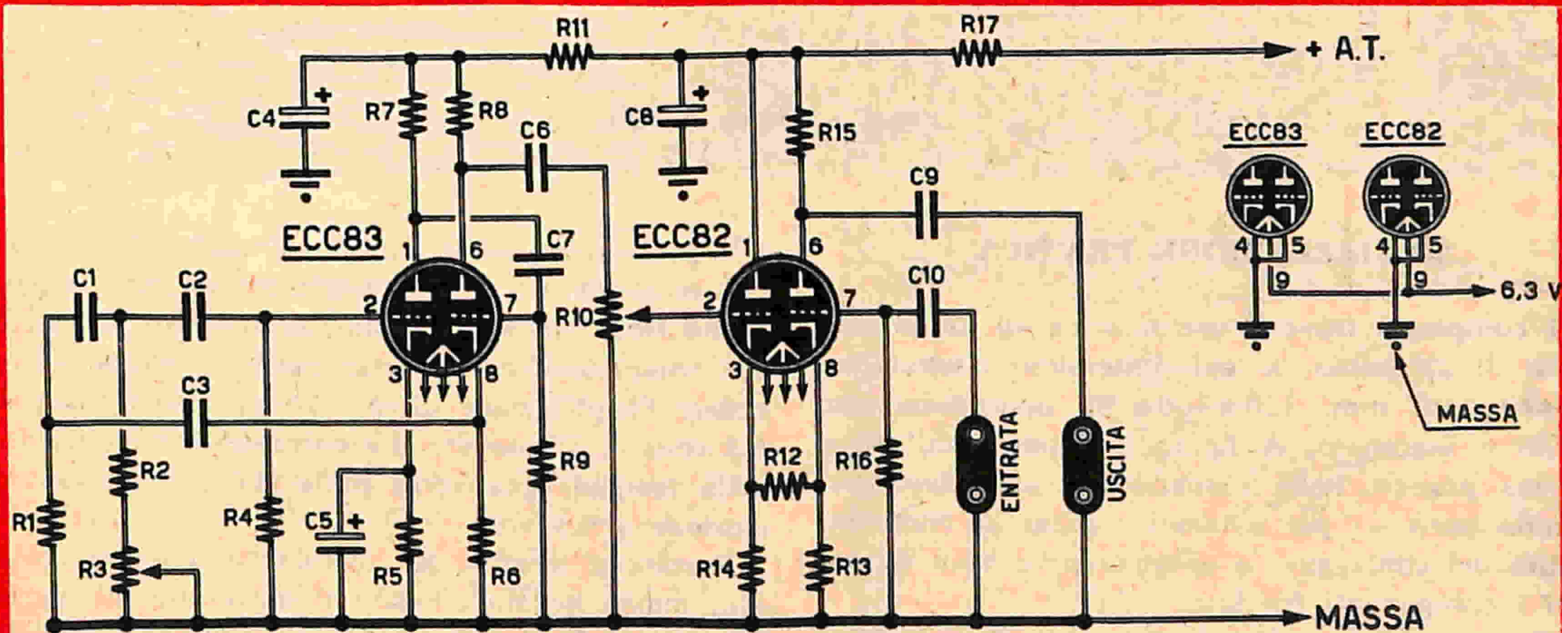
Fig. 1 - Schema elettrico ed elenco componenti.
