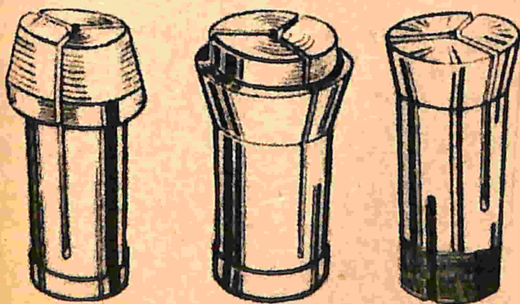
Fig. 3 - Pinze espansibili in nylon per pezzi lucidati o in materiali non ferrosi.
