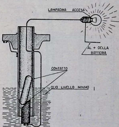
Fig. 2. — Quando l'olio comincia a scarseggiare, il galleggiante si adagia sul fondo, chiudendo il circuito.
