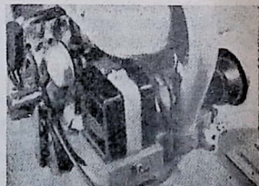
Fig. 3. - Nelle Lambrette C e D la soluzione migliore è quella di sistemare la batteria sotto il serbatoio della miscela.
