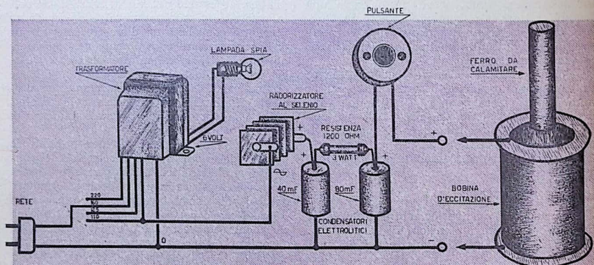
Fig. 2. — Schema pratico dell'alimentatore.
