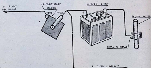
Fig. 1. - Schema pratico dell'impianto. Notare che per avere una buona presa di massa, il filo proveniente dal negativo della batteria dovrà essere collegato elettricamente al telaio, e pertanto il punto di contatto, dovrà essere preventivamente pulito da ogni traccia di vernice.
