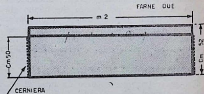
Fig. 2. — Parete verticale della tenda, cucito al telo principale per la parte superiore e fissato lateralmente con cerniere.
