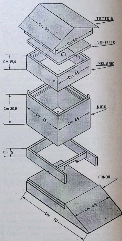
Fig. 2. - Parti principali che compongono l'arnia.
