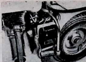
Fig. 4. - La batteria nella Lambretta E si dovrà invece sistemare sul fianco destro e precisamente tra il motore e la ruota posteriore.
