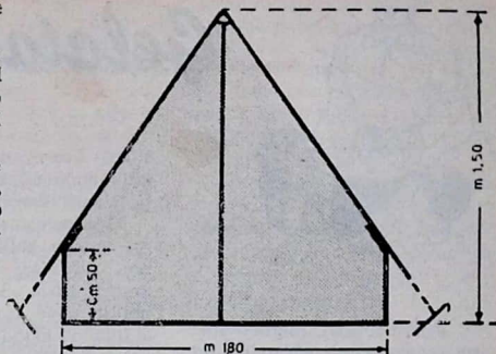
Fig. 4. — Schema della tenda vista di fronte.
