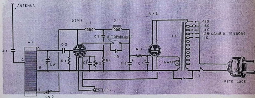
Fig. 1. - Schema elettrico
