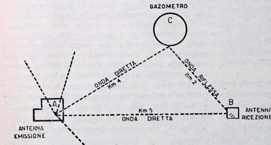
Fig. 5. — Schema di onda riflessa e differenza dei percorsi fra l'onda diretta e quella riflessa.
