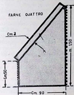
Fig. 3. — Forma di una mezza facciata con i vari sistemi da usarsi per fermarla agli altri vari pezzi della tenda.
