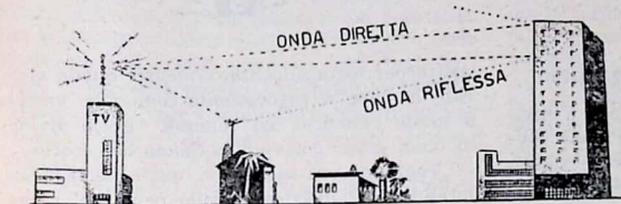
Fig. 4. — L'onda riflessa compie sempre un tragitto maggiore rispetto a quella diretta, perciò giunge sempre sullo schermo del televisore con un leggero ritardo, provocando lo sdoppiamento dell'immagine.
