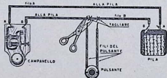
Fig. 1. - Installata la pila, si taglia un filo, collegando i due capi al pulsante.
