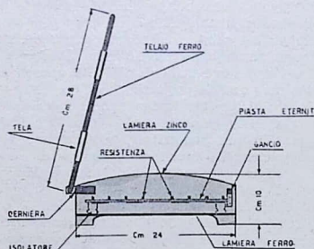
Fig. 1. — Smaltatrice vista di fianco.
