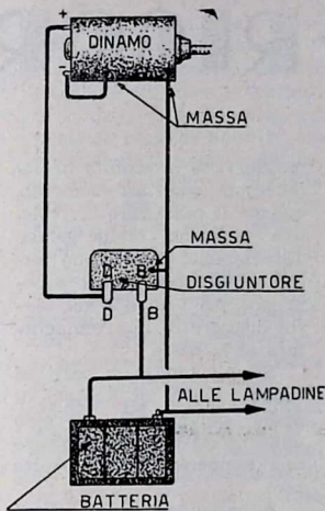
Fig. 5 - Schema elettrico del complesso.
