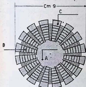
BOBINA A FONDO DI PANIERE
