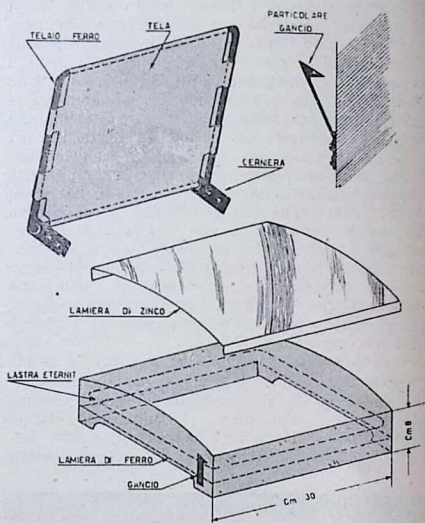
Fig. 2. — Vista dei vari pezzi componenti la smaltatrice.
