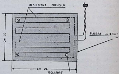
Fig. 3. — Disposizione della resistenza sulla piastra di Eternit.
