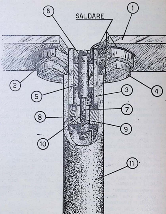
Fig. 4 - Particolare della spazzola, situata entro al tubo di sostegno.
