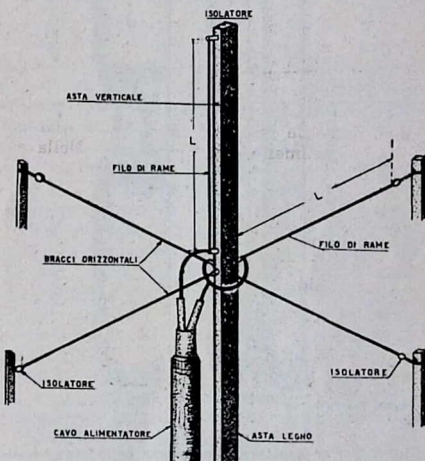
Fig. 2. - Quando non si ha la possibilità di usare tubi di alluminio, si può costruire la ground-plane utilizzando fili di rame e supporti di legno.
