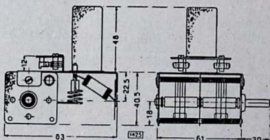
Le dimensioni di ingombro del gruppo N. 2693.
