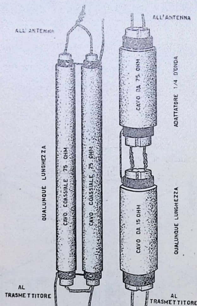
Fig. 3. - Per adattare l'impedenza della linea di alimentazione con quella dell'antenna, si possono utilizzare i due sistemi qui visibili. A sinistra abbiamo due cavi coassiali da 75 ohm collegati in parallelo. In questo caso 1 cavo può essere di qualunque lunghezza. A destra troviamo il sistema d'adattamento ad un quarto d'onda. Il cavo superiore da 75 ohm deve essere calcolato, di 1/4 d'onda mentre quello da 150 ohm può essere di qualunque lunghezza.
