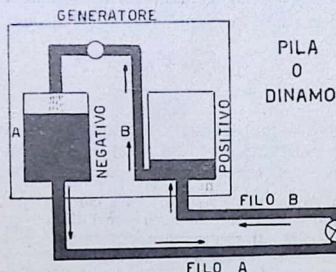
Fig. 1. - Corrente continua. Supponendo che A sia il polo negativo e B quello positivo di una pila e, ancora, che il generatore sia una pompa che aspira acqua da B per portarla in A. L'acqua, come la corrente continua, circolerà sempre in un senso.
