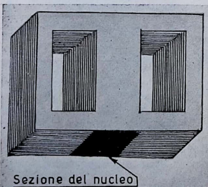
Fig. 1. - La sezione del nucleo si ottiene moltiplicando la larghezza della colonna centrale per lo spessore del pacco dei lamierini.
