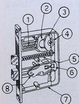
Fig. 1. - COMPONENTI: 1. Molla forcella - 2. Forcella - 3. Semidisco - 4. Mozzo - 5. Molla lucchetto - 6. Piastra oscillante - 7. Scatola - 8. Molla richiamo.
