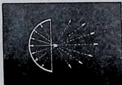
Fig. 4. — Riflettore sferico con lampada nel centro di curvatura. In queste condizioni i raggi si espandono su ad una superficie molto vasta, anche a breve distanze.
