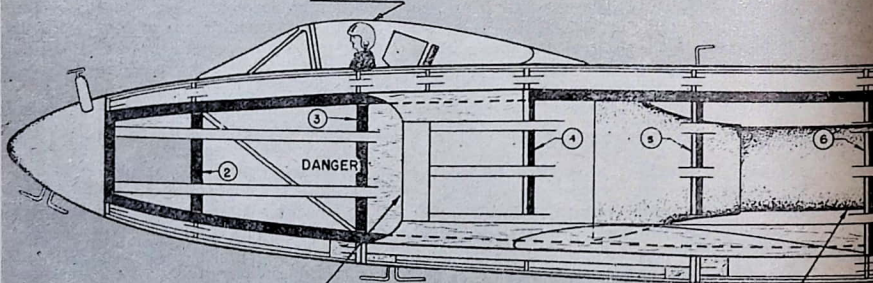
Vano per presa d'aria
