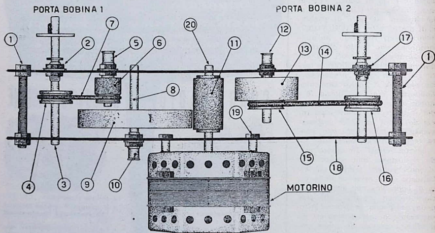
Fig. 1. - 1) Viti distanziatrici delle due lamiere. — 2) Boccola per il perno del PORTABOBINA 1. — 3) Perno, di 6 mm. di diametro, del PORTABOBINA 1. — 4) Rullo, con diametro di mm. 24, con scanalatura portante la cinghia di trasmissione. — 5) Perno di un vecchio potenziometro, diametro 6 mm. completo di boccola. — 6) Rullo di gomma con diametro di mm. 24 con scanalatura per la cinghia. — 7) Cinghia di trasmissione in gomma o a molla. — 8) (Vedi part. 5). — 9) Rullo di metallo di 85 mm. di diametro, altezza mm. 15, fissato sul perno 8. — 10) (Vedi part. 5). — 11) Rullo di gomma fissato al perno del motorino, diametro 16 mm. — 12) (Vedi part. 5). — 13) Rullo di metallo del diametro di mm. 45, spessore mm. 20. — 14) (Vedi part. 7). — 15) Rullo di metallo con scanalatura per cinghia, diametro: mm. 35. — 16) (Vedi part. 15). — 17) Boccola per il perno del PORTABOBINA 2. — 18) Piastra inferiore di metallo che sostiene il complesso. — 19) Viti che fissano il motorino al particolare 18.
