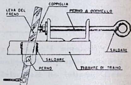
Fig. 2 - Posizione normale dell'impianto del freno.
