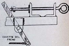
Fig. 2 - Posizione normale dell'impianto del freno.
