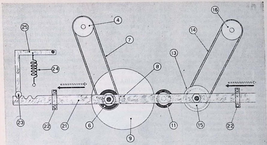
Fig. 2. - 4) Rullo di 24 mm. di diametro, sottostante il PORTABOBINA 1. — 6) Rullo di gomma fissato alla piastra n. 21, diametro mm. 24. — 7) Cinghia di trasmissione in gomma o molla. — 8) Perno con boccola, diametro, 6 mm. — 9) Rullo di metallo fissato al perno n. 8. — 11) Rullo del motorino. — 13) Rullo di metallo fissato al perno n. 12. — 14) (Vedi part. 7). — 15) Rullo di metallo con scanalatura. — 16) (Vedi part. 15). — 21) Asta metallica, spessore 2 mm., larghezza 15 mm. — 22) Guide metalliche per il part. 21. — 23) Rotella appartenente al dispositivo d'arresto, spessore mm. 5. — 24) Molla del dispositivo d'arresto. — 25) Leva azionante la rotella d'arresto. Il dispositivo d'arresto va fissato sullo stesso piano dell'asta mobile.
