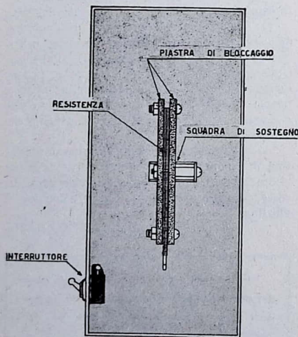
Fig. 1. — L'interno della stufetta, vista di fianco
