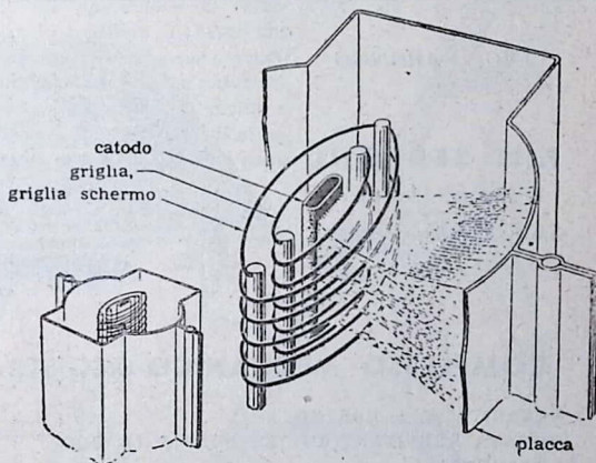
Fig. 3. - Rappresentazione dei vari elementi di una palvoia TE-TRODO, composta cioè di quattro elementi: CATODO, GRIGLIA, CONTROLLO, GRIGLIA SCHERMO, PLACCA. Si notino le griglie costruite con spirali di filo in modo che gli elettroni possano passare attraverso gli spazi e raggiungere la placca.
