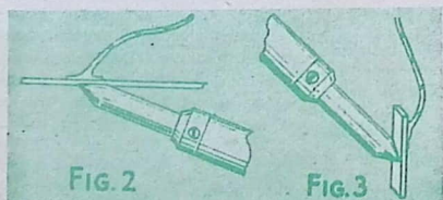
FIG. 2. — Come va effettuata una saldatura orizzontale. FIG. 3. — Come invece su di un piano verticale.
