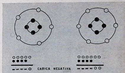
Fig. 3. - Ecco due atomi che per avere il numero degli elettroni superiore a quello dei protoni si trovano caricati di elettricità NEGATIVA .
