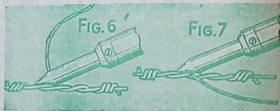
FIG. 6. — Modo errato di sciogliere lo stagno. FIG. 7. — Come lo stagno va sciolto: cioè sul pezzo da stagnare e non sul saldatore, come avviene, invece, in fig. 6.
