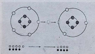
Fig. 5. - L'atomo di sinistra carico negativamente tenderà a cedere un elettrone all'atomo positivo neutralizzando così la sua carica.
