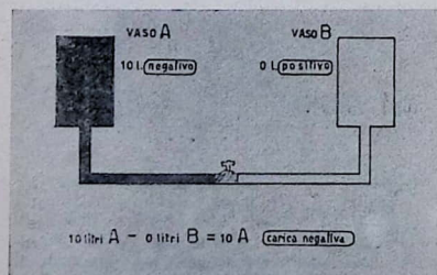
Fig. 6. - Siano A e B due atomi carichi di elettricità di segno contrario.
