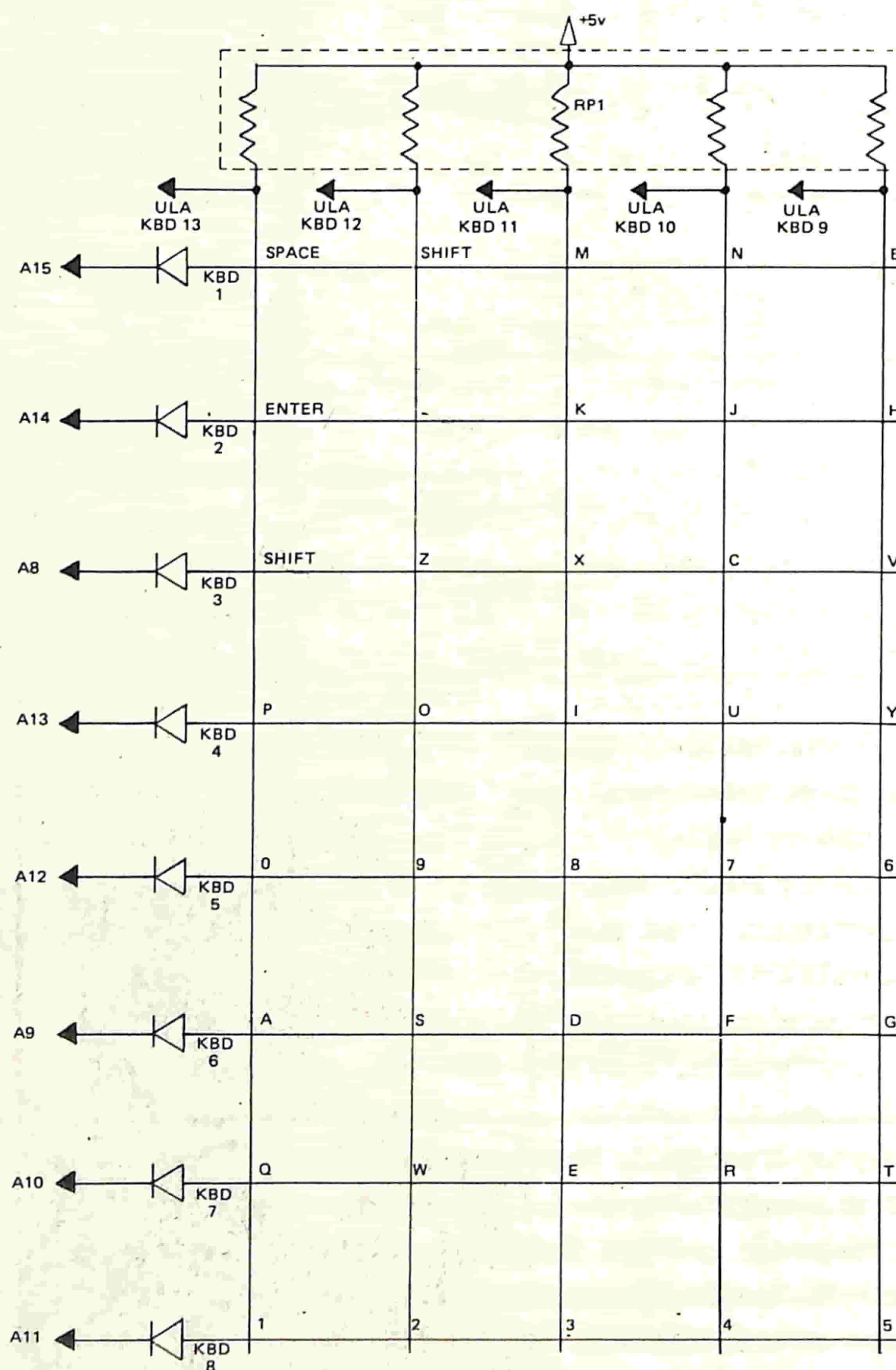
Fig. 5. La tastiera dello Spectrum: lo schema logico.
