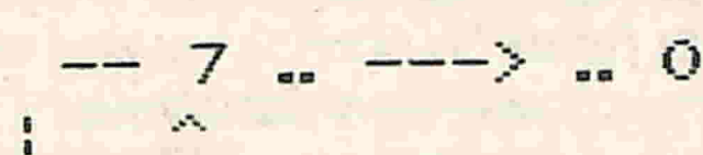
fig. 7 - Spostamento logico a destra (SRL)
