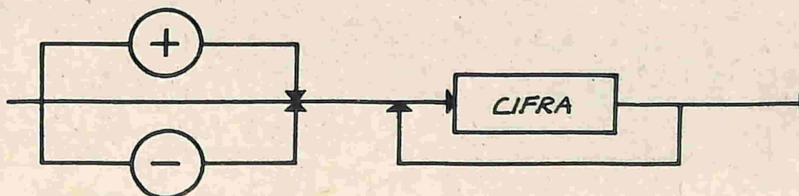
FIG. 2 - NUMERO INTERO
