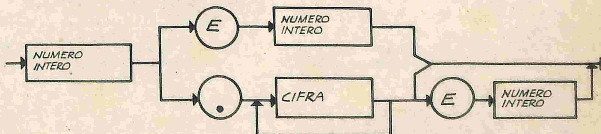
FIG. 3 - NUMERO REALE
