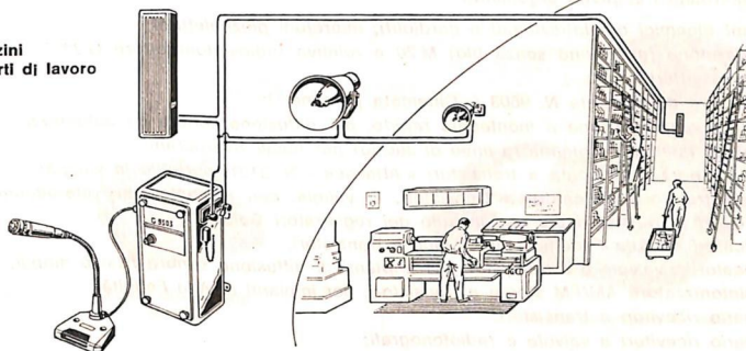
Due altoparlanti a colonna N. 3109 e due trombe esponenziali N. 2570.
