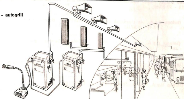
Impianto con due amplificatori 9503, uno per l'interno con quattro colonne N. 3109, l'altro per l'esterno con quattro trombe N. 2537/2531.
