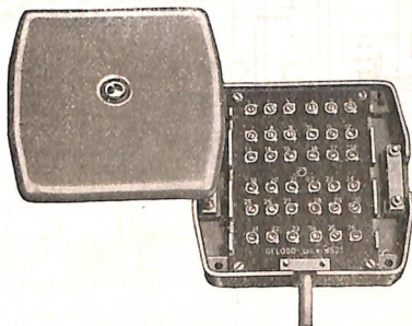
Morsettiere di derivazione N. 9521.
