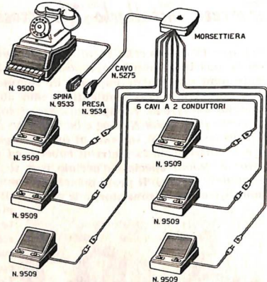
Impianto interfonico costituito da un posto di comando 9500 collegato con sei posti dipendenti 9509
