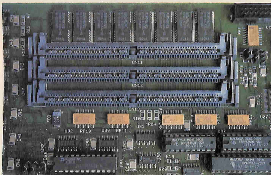
La Ram aggiuntiva montata sulla scheda GVP Impact (1 oppure 4 Mb), e gli slot Simm che possono contenerne altri 12 Megabyte.
