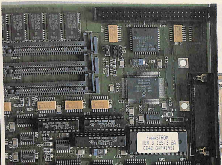
I connettori esterno e interno del controller SCSI compreso nella Gvp Impact Serie II, in grado di pilotare fino a 7 periferiche.
