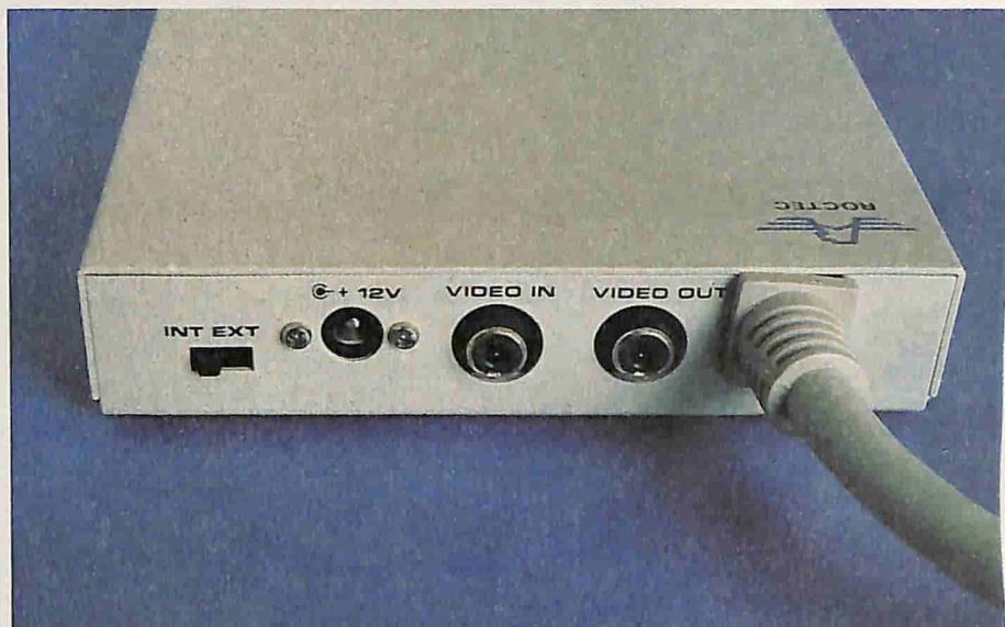
I connettori di input/output del genlock Rocgen.
