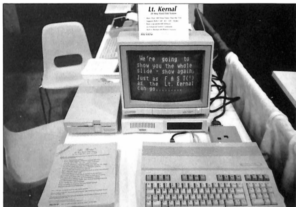
L'Amiga collegato al Sidecar
