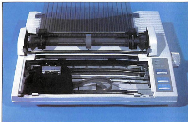
In alto: notare il paper bail, il trattore ed il separatore di fogli. In basso: prova di stampa. Notare i vari modi di scrittura ed in particolare quello NLQ.
