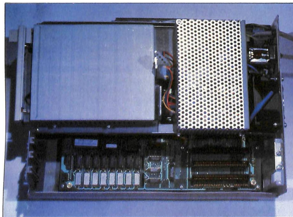
In alto: la scheda madre. In basso: l'interno del Sidecar
