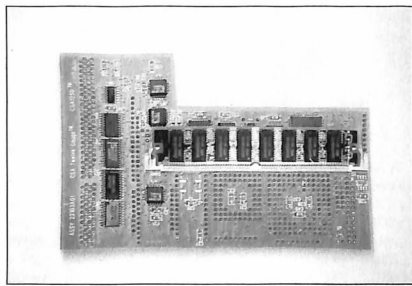
Il lato con la CPU (sopra) della scheda Twelve Gauge della CSA e il suo cavo SCSI. Il lato SIMM (sotto) della stessa scheda
