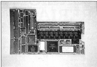
La scheda SCSI/RAM+ realizzata dalla Great Valley Products
