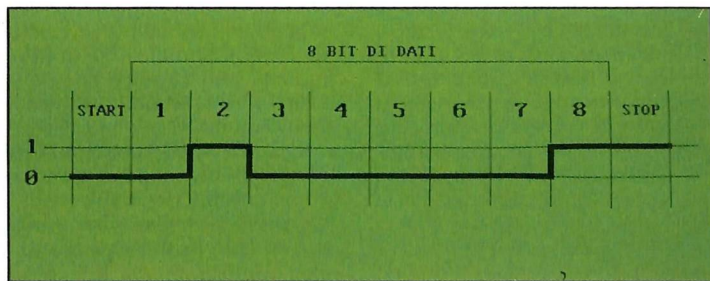
Il diagramma mostra l'invio della lettera "e" con 8 bit e nessun bit di parità
