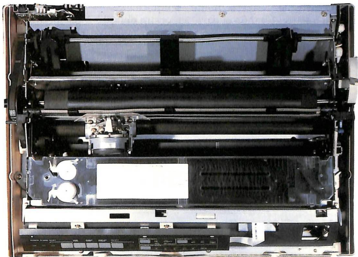
L'esame interno rivela solidità costruttiva. Si noti il capace caricatore d'inchiostro
