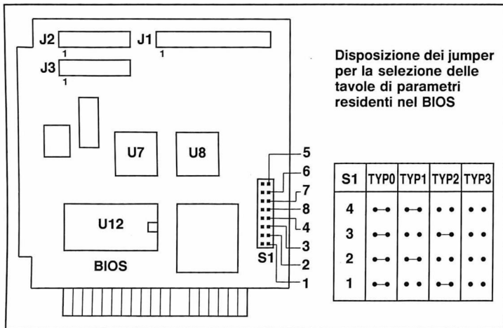
Le configurazioni dei jumper del controller PC 5060 per la selezione dei parametri
