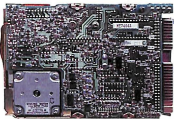
Il circuito di controllo del disco rigido
