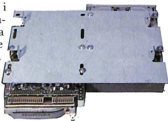
L'hard disk a fianco del drive df0:
