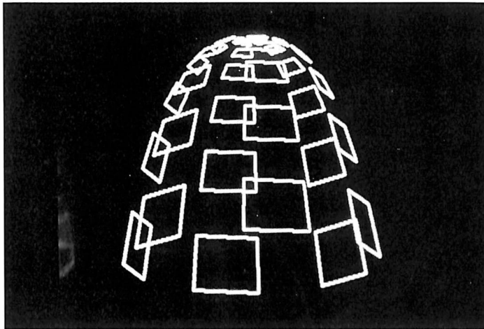
Sopra: rappresentazione "a quadrati" della funzione XX=U*\sin(V) ; YY=U*\cos(V) ; ZZ=(U*U)*\sqrt{U*U}/10 , e i limiti UI=1 , US=2 , VI=0 , VS=6.28 . Sotto: particolare della figura di pagina 104, ottenuto variando i limiti dei parametri
