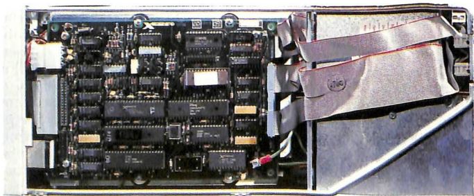
Visione completa del circuito e del cablaggio interno dell'hard disk 9740H della Xebec
