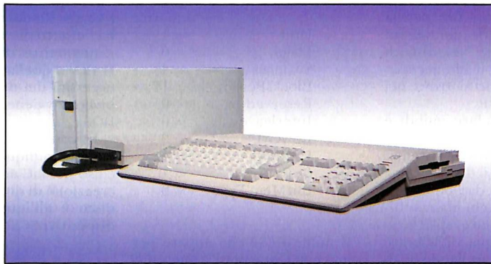
L'hard disk Xebec collegato tramite interfaccia al connettore sinistro dell'Amiga 500
