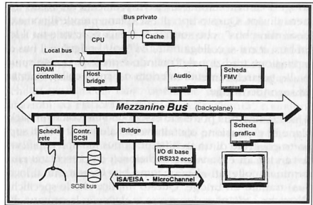
Figura 1 - Architettura dei personal computer con mezzanine bus.
