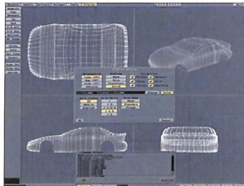
Fig. 2 - LightWave 3D/Modeler. L'editor aperto in 1.192x900 su Picasso II. I pesanti problemi di compatibilità che affliggevano la revisione 3.5 sono stati risolti. Nella figura appaiono i requester di tipo ASL di sistema impiegati al posto dei precedenti e la scelta interna e diretta della risoluzione grafica di apertura.
