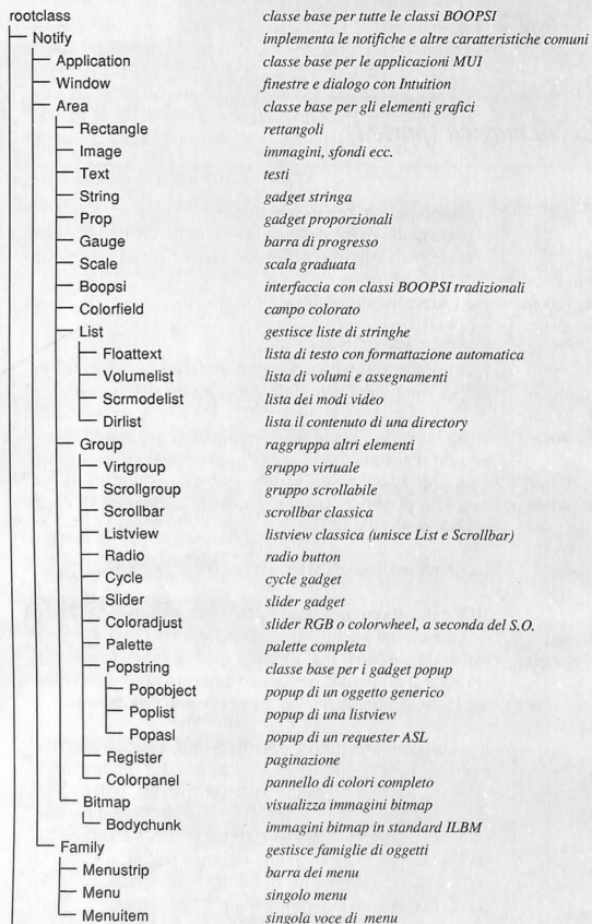
Fig. 1 - L'albero delle classi di MUI.
