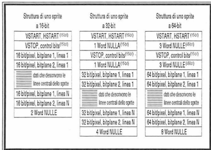
Figura 2 - I tre tipi di sprite presenti sotto AGA.
