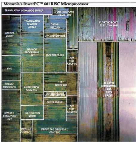
Fotografia del chip MPC601 visto al microscopio polarizzatore. Sono evidenziati i sottosistemi principali. Immagine fornita da Motorola, inc.
