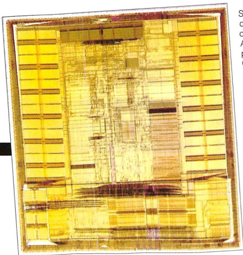
Il microprocessore Digital Alpha 21164, il più potente tra quelli in commercio. Consuma 50 W e richiede un impianto di raffreddamento dedicato.
