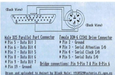
Fig. 1 - Cavetto Amiga - seriale Commodore.
