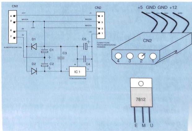
Fig. 2 - Adattatore per usare l'alimentatore C64 con periferiche standard.
