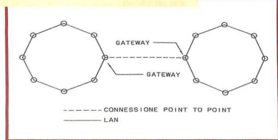
Fig. 2 - Due LAN interconnesse tra loro per formare una WAN. Si vedono le due macchine con ruolo di gateway, ossia in grado di gestire l'interscambio di dati tra le due LAN.
