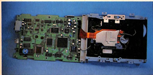
NEC CDR201 aperto.
