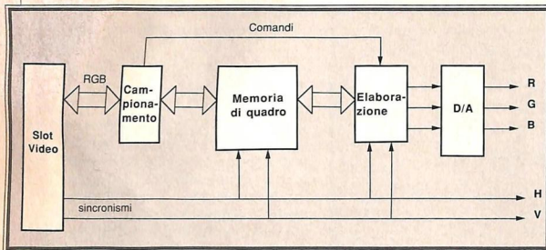
Fig. 3 - Schema a blocchi delle schede per slot video con memoria di quadro.
