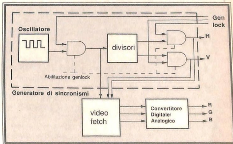
Fig. 1 - Schema a blocchi del circuito di generazione sincronismi e pilotaggio monitor.
