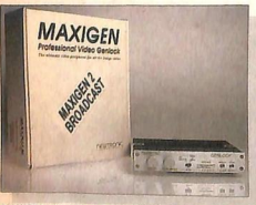
MAXIGEN. Genlock Broadcast VHS e S-VHS, regolazione del livello di saturazione in ingresso. Superimpose, FADE professionale, Invert Key, porta RGB passante, Cromo Key, nove regolazioni accessibili esternamente. Banda passante 5,7 Mhz - 3Db.
