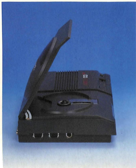
I connettori laterali del CD32: porte joystick e Aux per tastiera.
