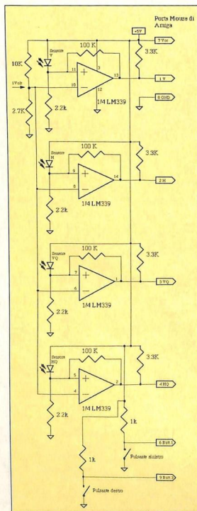
Schema elettrico del circuito che genera i segnali necessari ad Amiga. Normalmente si trova già nel mouse.
