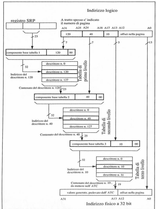
Figura 2: Traslazione effettuata da una MMU del 68040, nel caso in cui tutte le tabelle vengano consultate. Dopo la ricerca in memoria, la parte più significativa dell'indirizzo fisico viene posta nell'ATC.
