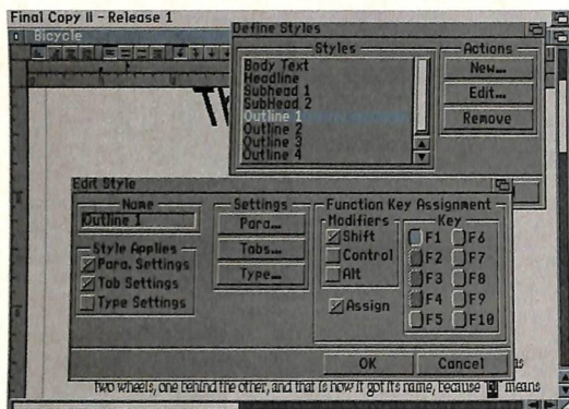
Pannello per l'impostazione degli stili.
