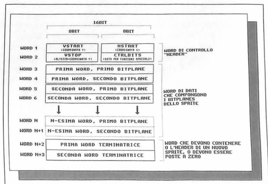
Figura 2: Struttura sprite
