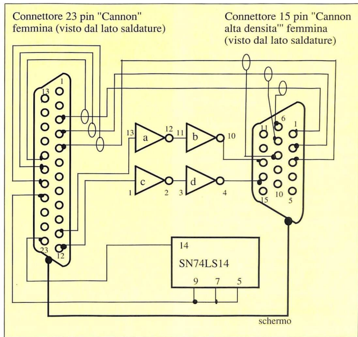
Figura 2: Adattatore Amiga RGB-> VGA completo. I conduttori dei segnali R, G, B (pin 1, 2, 3 del connettore VGA) sono schermati; la calza va saldata sui pin 6, 7, 8; a, b, c, d sono inverter contenuti nel circuito integrato SN74LS14.
