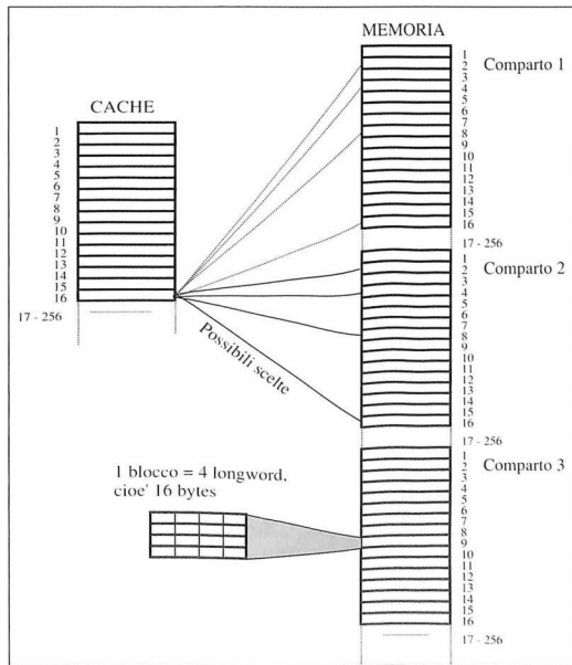
Figura 3: Schema di una cache 4 way set associativa (68040)
