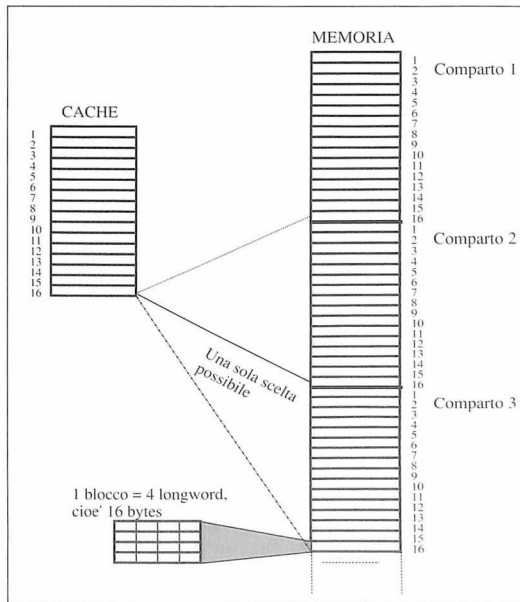
Figura 4: Schema di una cache direct mapped (68030)
