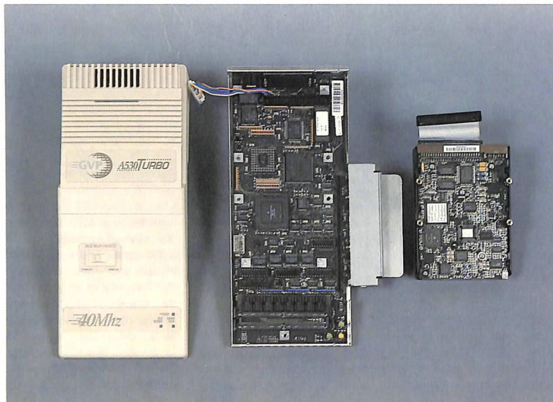
L'interno della A530.
