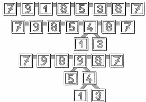
Figura 2: Costruzione dell'albero di Huffman a partire dalla lista di nodi delle frequenze.
