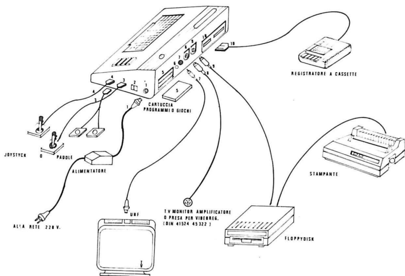
FIG.4. Schema di alcune delle periferiche collegabili direttamente al sistema
