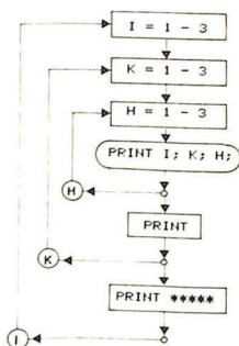
FIG.13. Schema a blocchi di cicli for next nidificati
