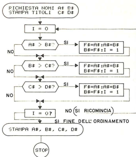
FIG.9. Schema di ordinamento tra stringhe (SORT)
