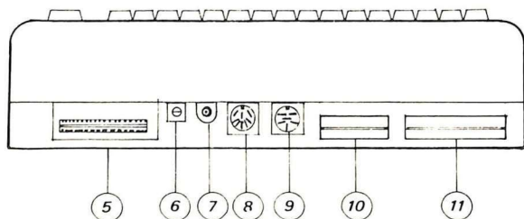
FIG.3. Vista posteriore con prese per connessioni varie
