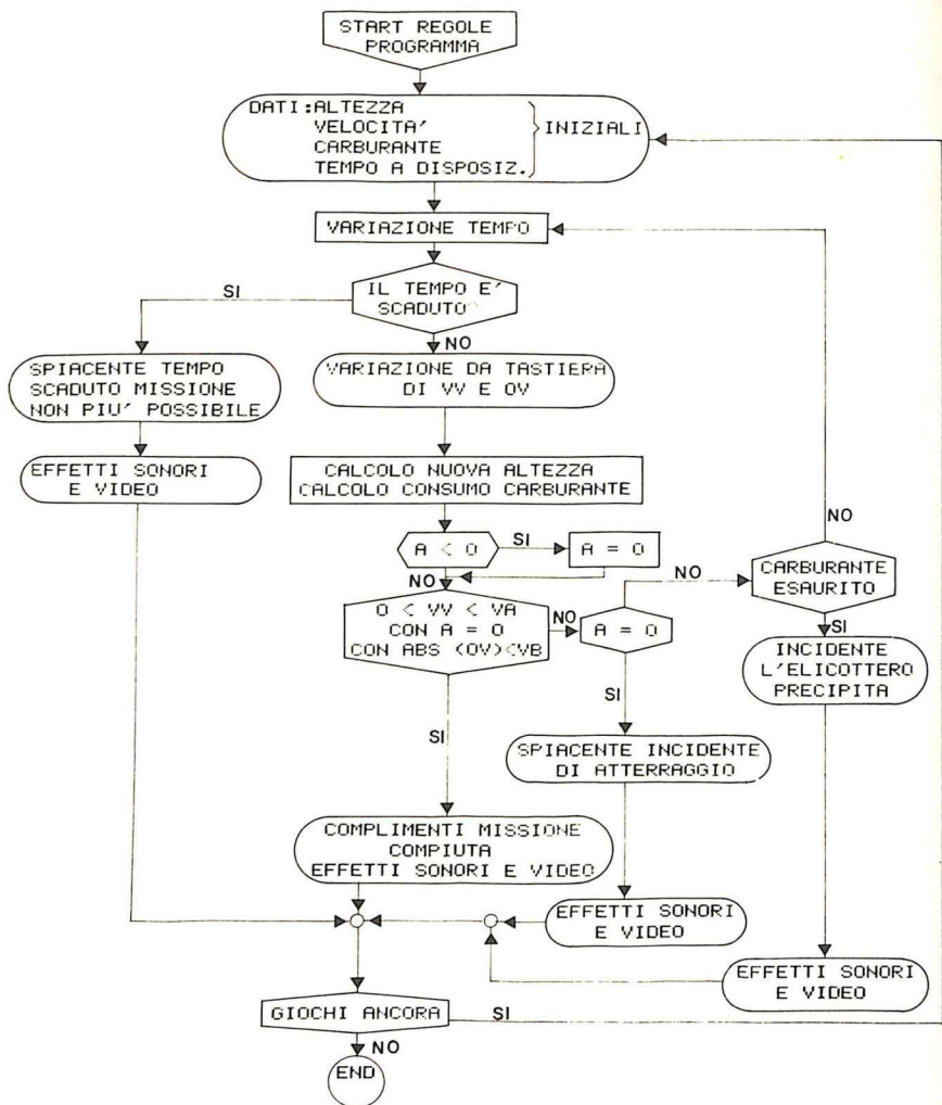
FIG.12. Schema a blocchi programma elicottero
