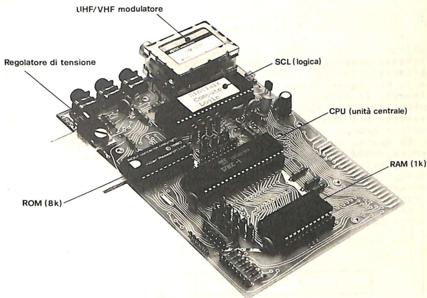
Fig. 2.2. Il calcolatore ZX81 aperto
