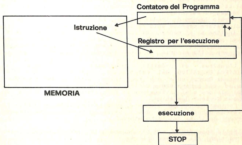
Fig. 2.5. Schema dell'automatismo
