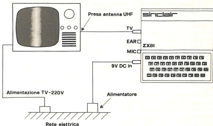
Fig. 3.5. Schema di collegamento per lo ZX81
