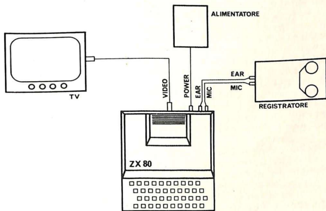
Fig. 3.1. Schema di collegamento per lo ZX80
