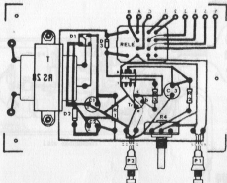
lato componenti
