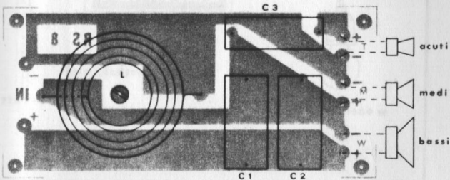
Lato componenti
