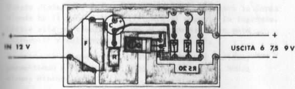
Lato componenti
