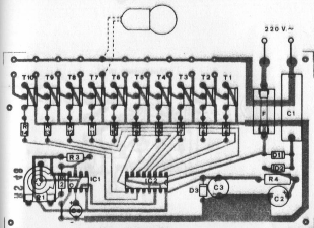
Lato componenti
