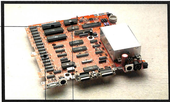
Figura 3-1. La scheda logica principale
