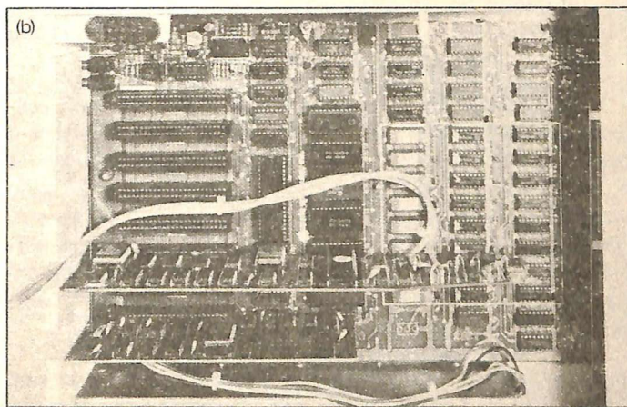
Fig. 5.3 (a) L'interno dell'Apple II (b) l'interno mostra la cartolina di interfaccia
