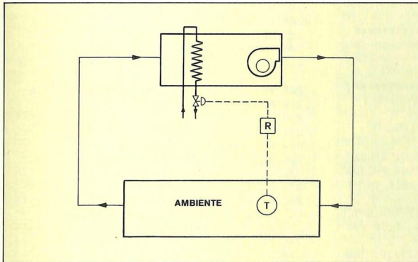
Figura 5 - La rappresentazione dell'impianto.
