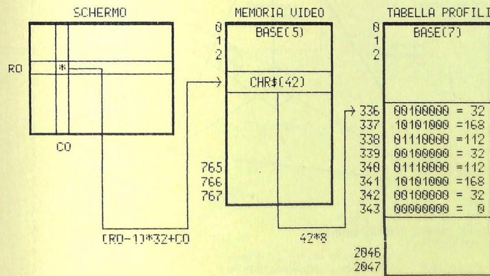
Figura 6 - Nel modo testo 2 la mappa di memoria del video è più limitata. In compenso i simboli grafici vengono visualizzati in modo più completo ed esiste una maggiore libertà nell'uso dei colori, in virtù di una tabella di memoria non riprodotta nella figura.
