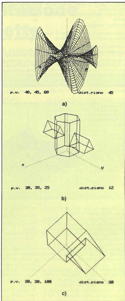
Figura 8a,b,c - Alcuni disegni ottenuti con il programma.
