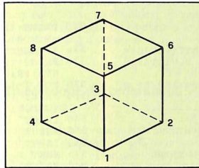
Figura 6 - Numerazione degli 8 vertici di un cubo.
