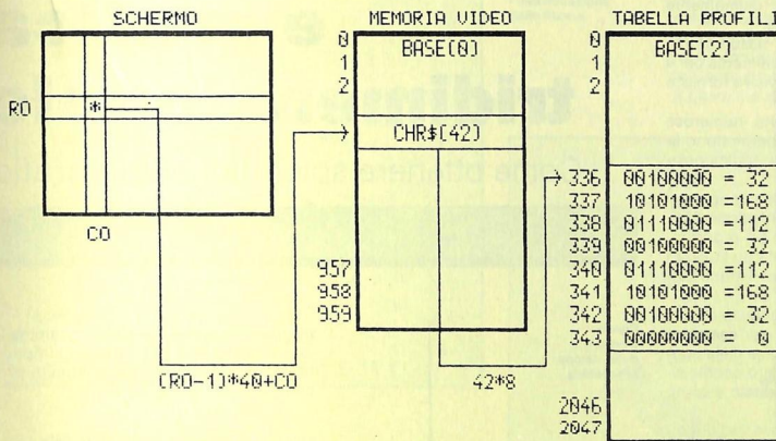
Figura 5 - Le parti più importanti della VDP RAM sono la mappa di memoria del video e la tabella dei profili, cioè delle forme dei caratteri. Ogni elemento della mappa contiene il numero di codice ASCII del carattere presente in una data posizione dello schermo e ad ogni carattere corrisponde una sequenza di 8 byte nella tabella dei profili.
