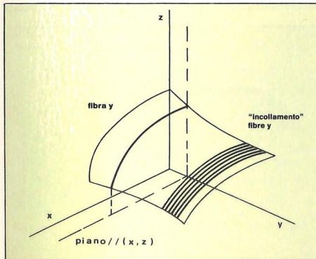
Figura 3a,b,c - incollamento della fibra x, y ed r.
