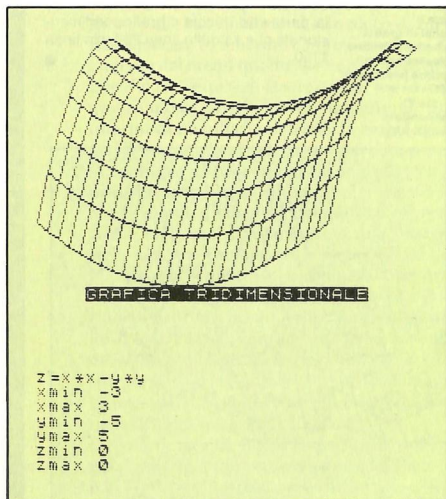
Figura 2 - Esempio di utilizzo del programma: la figura ottenuta è un parabole a sella.
