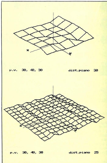
Figura 4a,b - Rappresentazione di valori di quota utilizzando un reticolo x,y .
