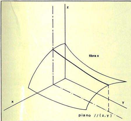
Figura 2 - Rappresentazione di superfici funzionali mediante l'individuazione delle fibre x.
