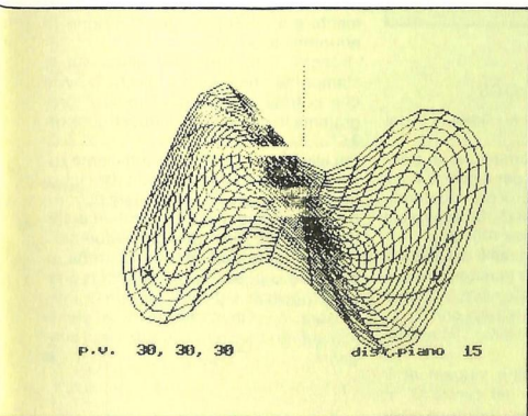
Figura 7 - Rappresentazione d'una funzione con diverse modalità.
