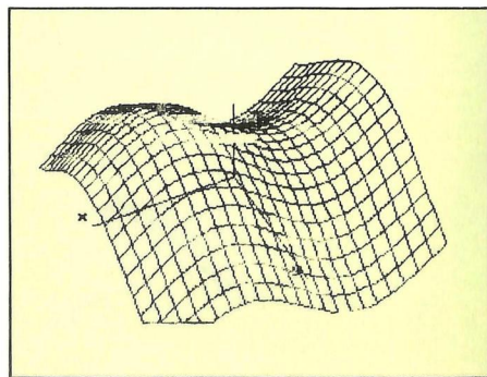
Figura 5 - Funzione empirica approssimante una più complessa
