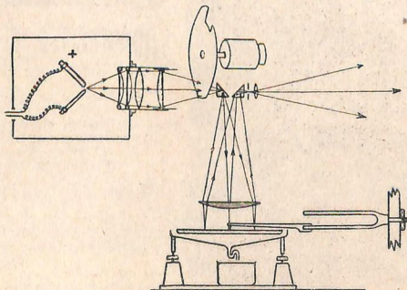
Fig. 7. - Disegno schematico dell'Ondoscopio.
