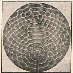
Fig. 6. - Riflessioni ellittiche.
