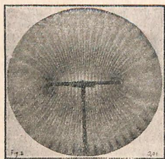
Fig. 2. - Con due punti vibranti si ha questo sistema di onde (luce continua).
