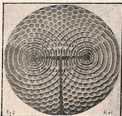
Fig. 3. - Come la fig. 2, ma a luce intermittente, appare chiaramente il vero modo di interferire dei due sistemi di onde.
