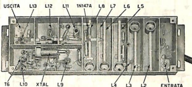
Vista superiore ed inferiore del convertitore G 4/163, coi punti di taratura. Top and bottom views of G 4/163 converter, with alignment points.
