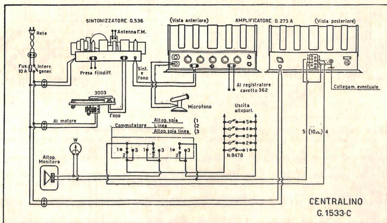
Schema generale del G 1533-C
