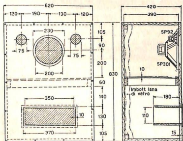
Fig. 2 - Altro modello di mobile « bass-reflex ». Pareti in legno d'abete, spessore \text{cm } 1,5 \div 2 . L'imbottitura, da farsi sulla sola parete di fondo, è formata con lana di vetro com'è detto per il mobile della fig. 1. Il mobile è diviso all'interno in due parti uguali mediante un diaframma di materiale fonoassorbente forato (con 100 fori \varnothing 3 \text{ mm} per decimetro quadrato). Tale diaframma potrà essere richiesto a qualche ditta che tratta materiali di questo genere (la nostra Casa per ragioni di correttezza non dà indirizzi). La finestra inferiore è munita di una appendice tubolare di sezione rettangolare posta all'interno del mobile, come mostra la figura, e chiusa nella parte esterna con un diaframma di materiale fonoassorbente forato come il diaframma mediano interno.
