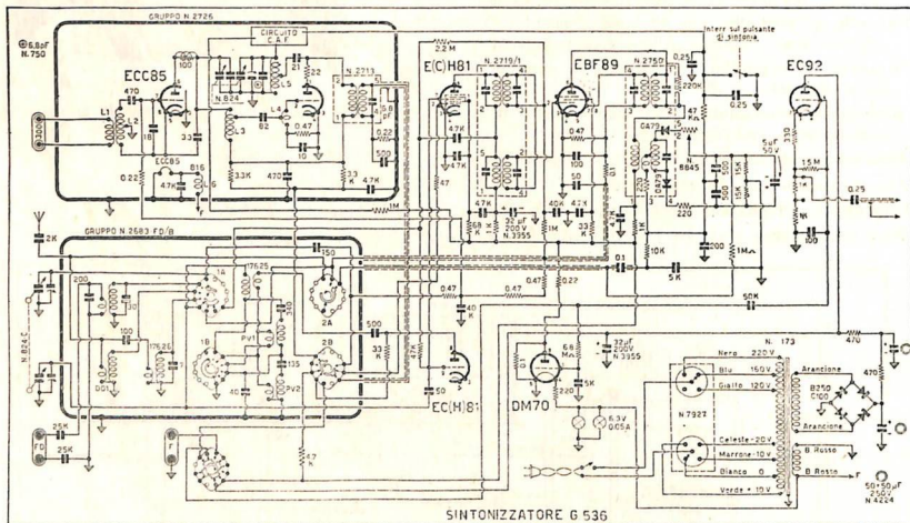
SINTONIZZATORE G 536
