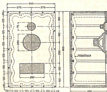
Fig. 1 - Mobile diffusore « bass-reflex ». E costruito in legno d'abete ben stagionato: spessore 2 \div 3 \text{ cm} . Sul fondo e sulle pareti laterali, all'interno, sono fissati listelli di legno (incollati e inchiodati) come mostra la figura. Su tali listelli è disteso, in modo da risultare ondulato, uno strato di lana di vetro (spessore 3 \div 4 \text{ cm} ) oppure di altra materia equivalente, tenuto a posto mediante uno strato di garza o di velo e chiodi piantati non a fondo tra un listello e l'altro. La parete interna frontale non è imbottita.
