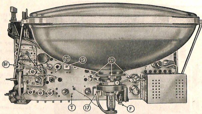
Fig. 9 - GTV 1035. Telaio visto di sopra.
