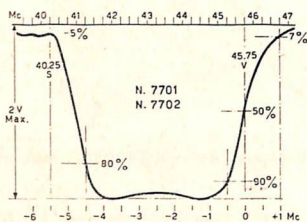
Fig. 15 - Fac simile della curva di risposta delle sezioni a FI N. 7701 e N. 7702 (nei televisori GTV 1044 e GTV 1045).
