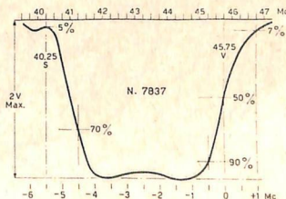
Fig. 14 - Fac-simile della curva di risposta della sezione FI N. 7837 (nei televisori GTV 1010 e GTV 1035).
