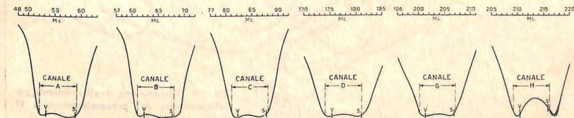
Fig. 21 - Fac-simile delle curve di risposta più caratteristiche dei sintonizzatori VHF N. 7870 e N. 7871.
