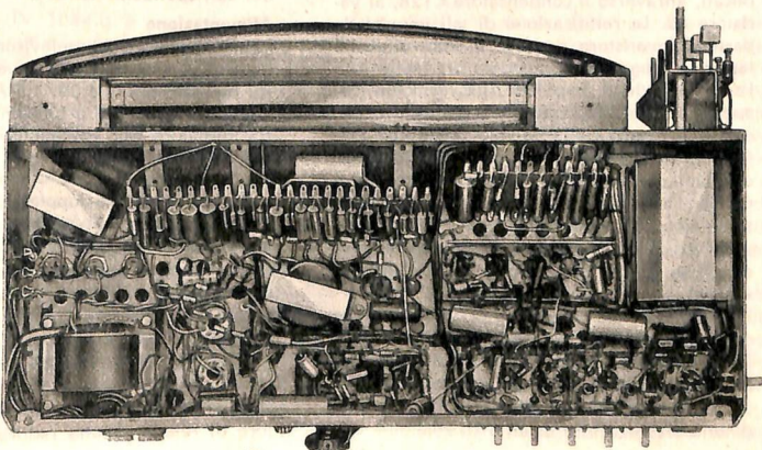
Fig. 4 - GTV 1045. Telaio visto di sotto.
