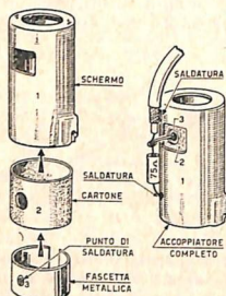
Fig. 12 - Accoppiatore capacitivo per la valvola miscelatrice ottenuto con uno schermo per « novel » convenientemente adattato:
