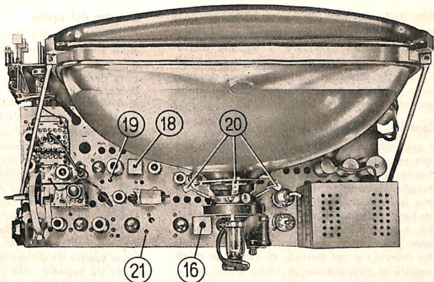
Fig. 3 - GTV 1045. Telaio visto di sopra.
