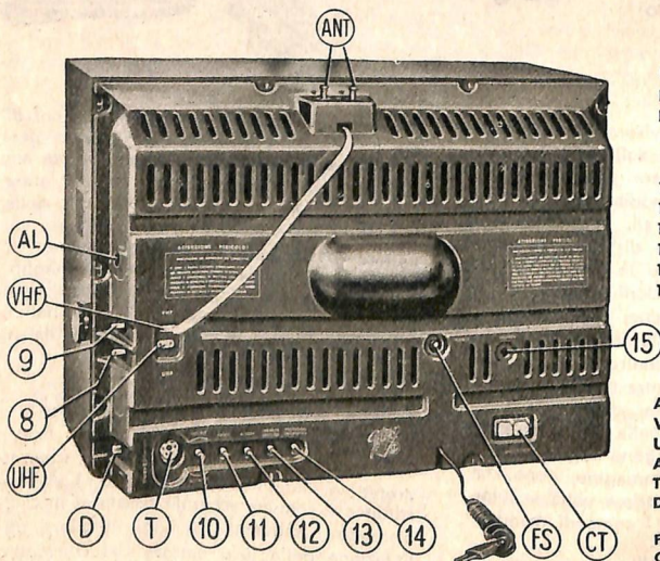
Fig. 2 - GTV 1045. Organi, prese e comandi laterali e posteriori.
